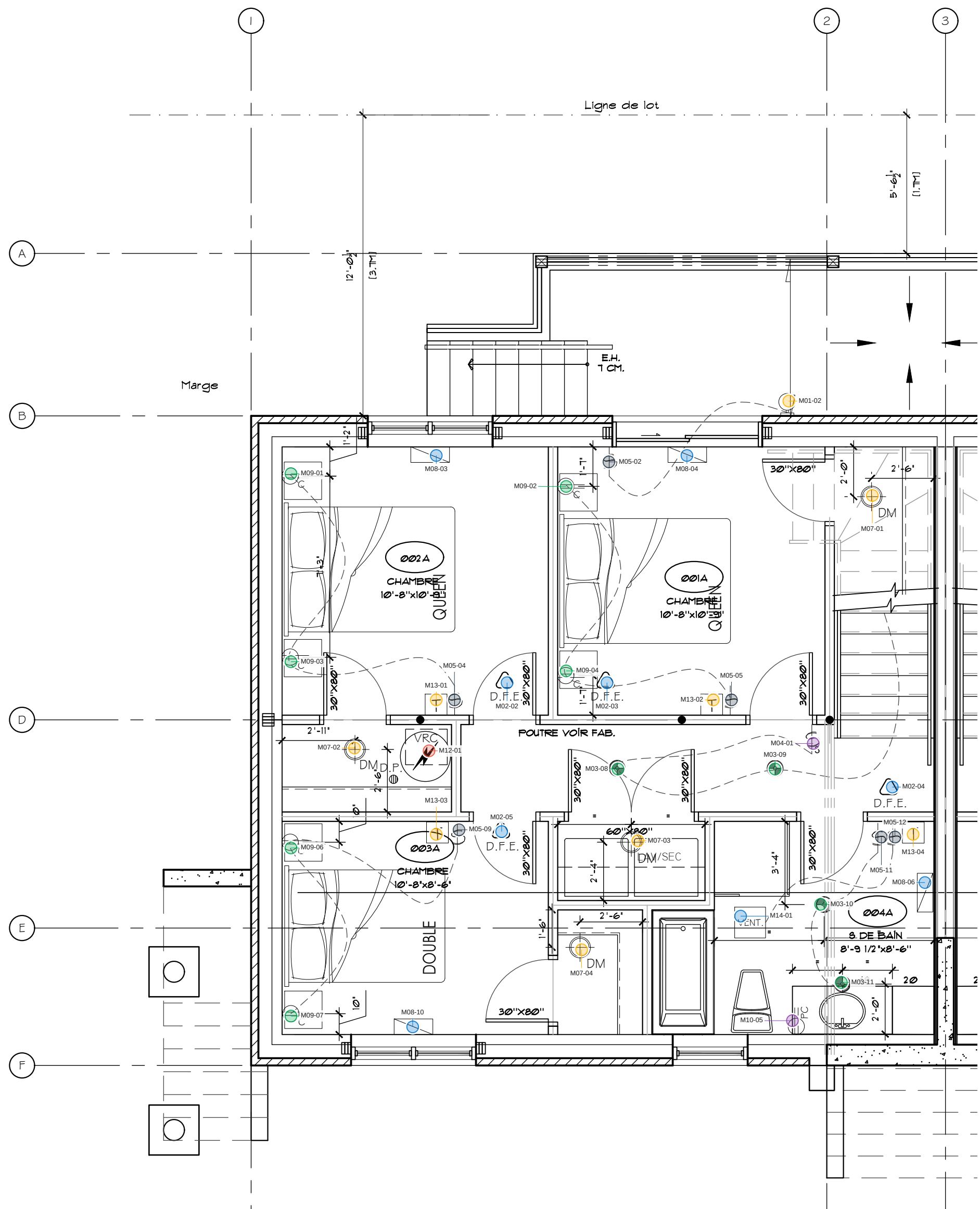
UNITÉ TYPE A - PLAN SOUS-SOL NOUVELLE CONDITION Echelle 1/4" = 1'-0" A-801
