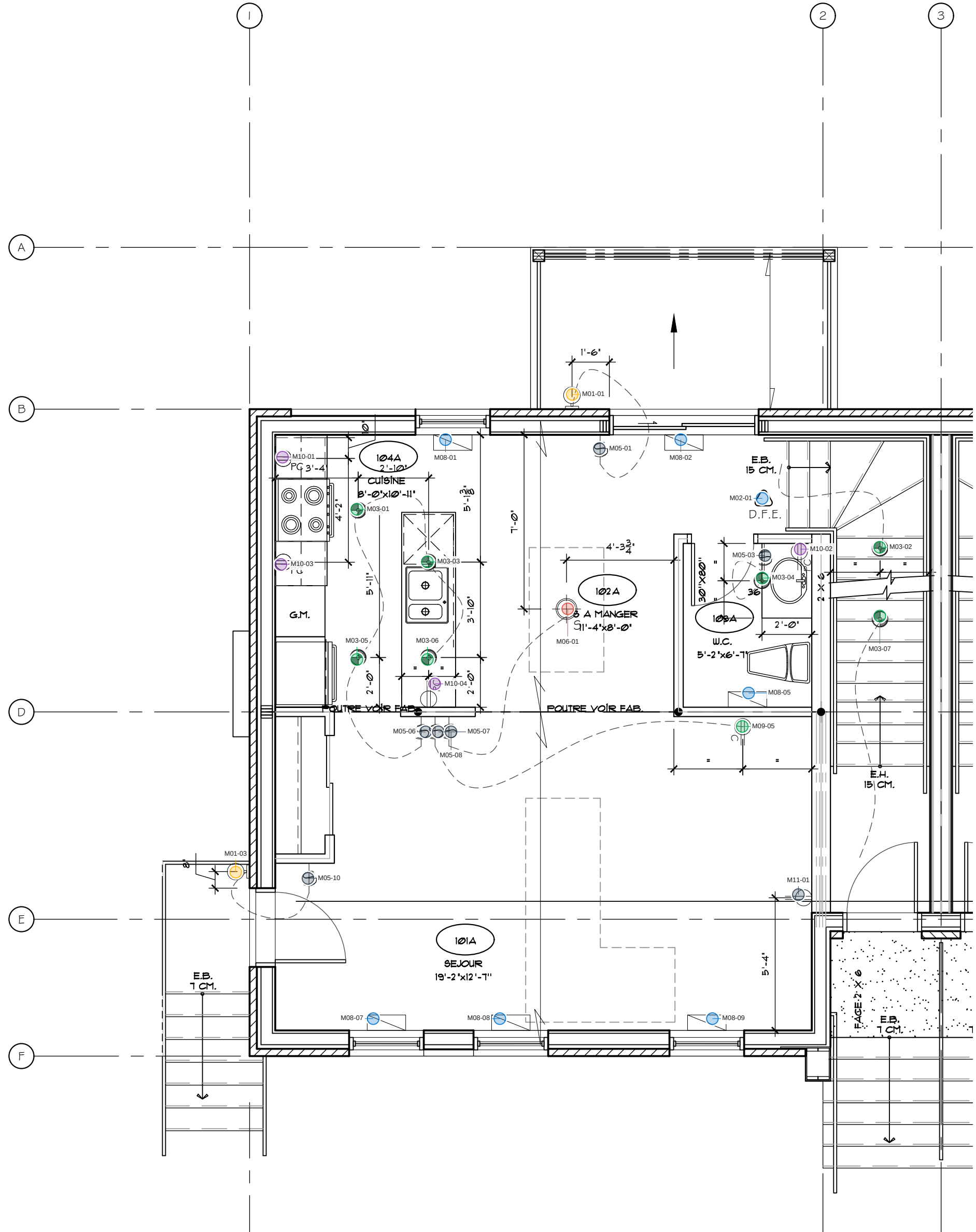
UNITÉ TYPE A - PLAN DU REZ-DE-CHAUSSEE NOUVELLE CONDITION Echelle 1/4" = 1'-0" A-801
