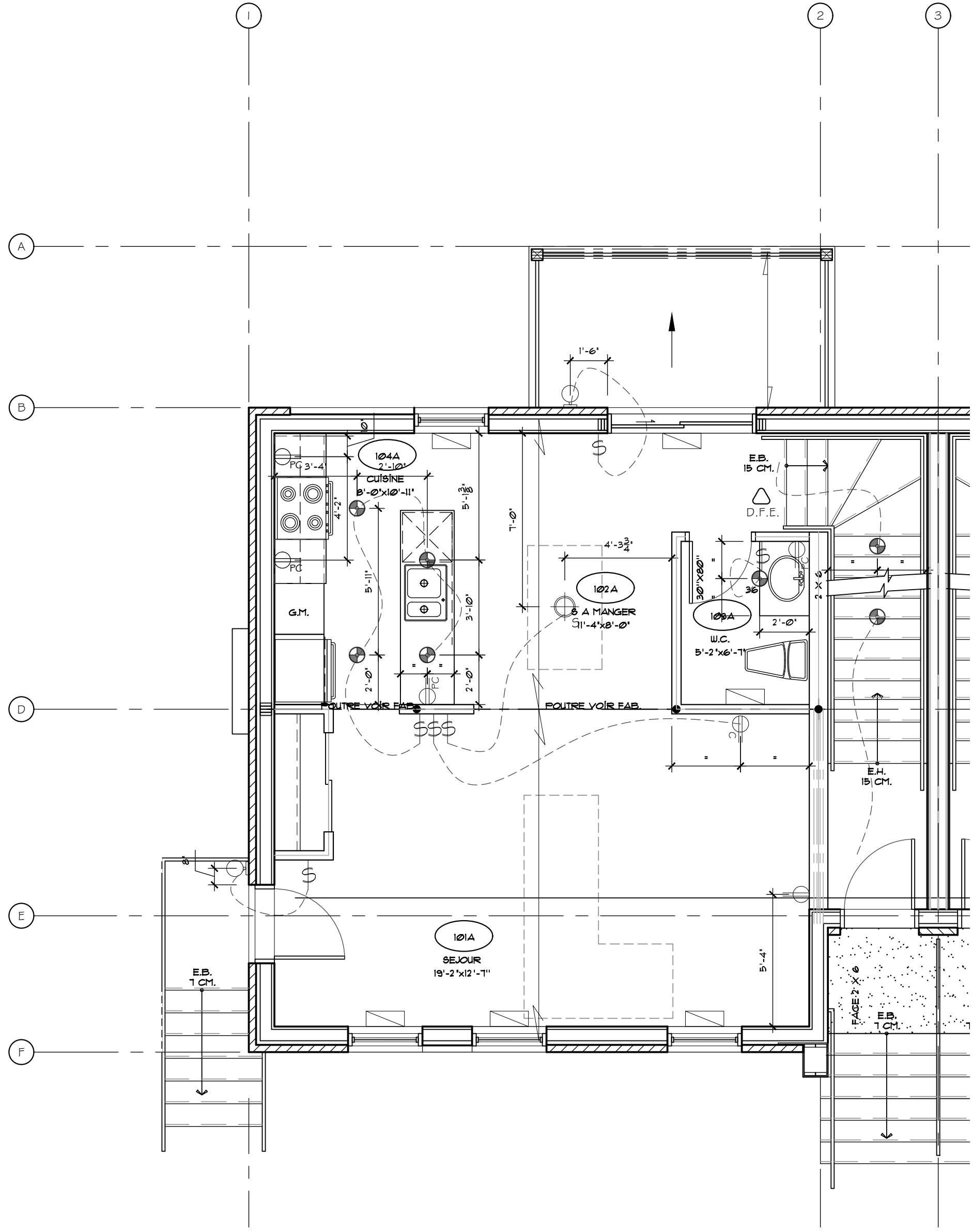
UNITÉ TYPE A - PLAN DU REZ-DE-CHAUSSEE NOUVELLE CONDITION ÉCHELLE 1/4"=1'-0" A-801
