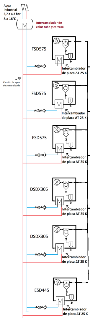
Figura 1: Esquema del sistema de recuperación de calor propuesto.
