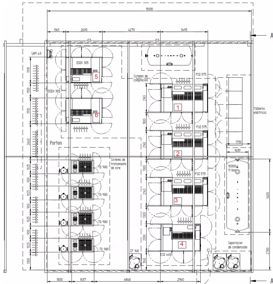
Figura 2: Plano de distribución de los compresores en la sala de máquinas.
