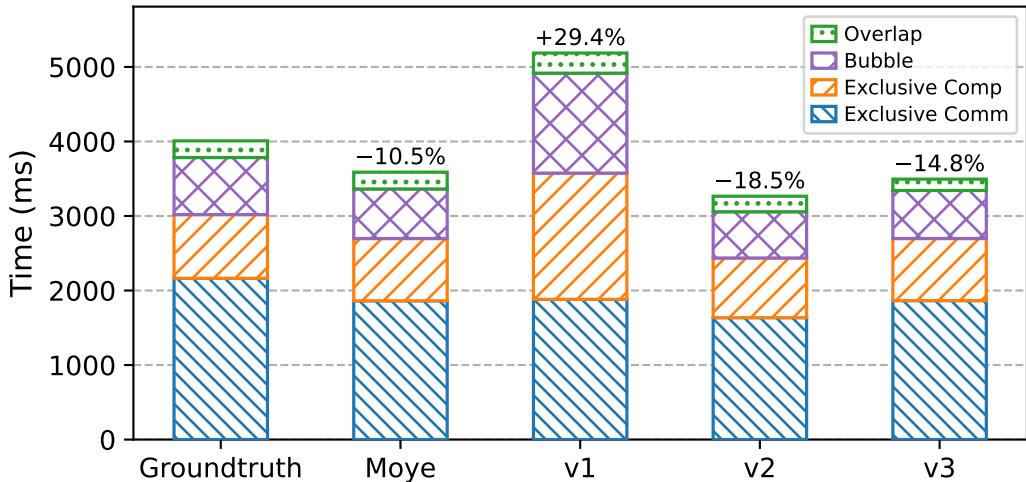
E2E Components Breakdown (H800-256GPUs-GPT175B)
