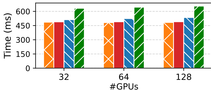
GPT2
