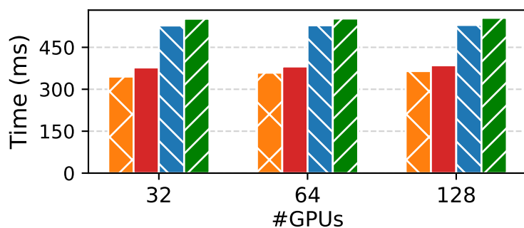
GPT2
