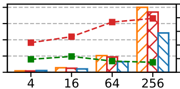
AllGather
