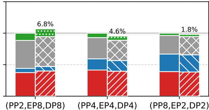
Qwen3-A3B
