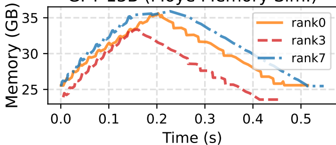
GPT 13B (Moye Memory Sim.)
