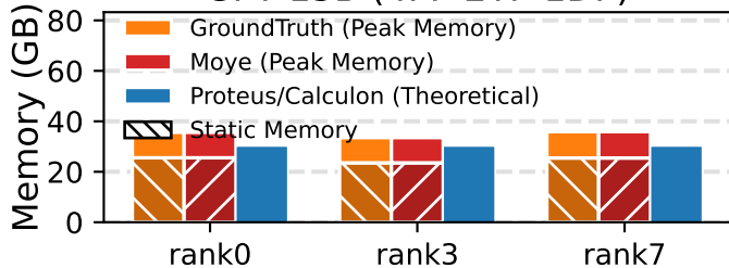
GPT 13B (Moye Memory Sim.)
