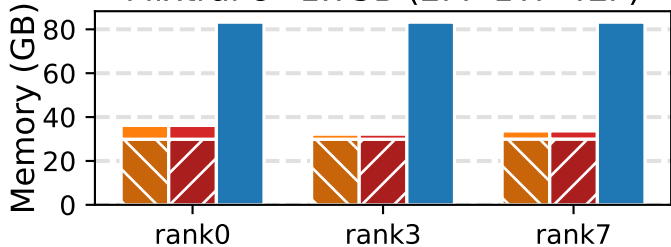
Mixtral 8×1.75B (Moye Memory Sim.)
