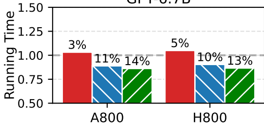
GPT-6.7B
