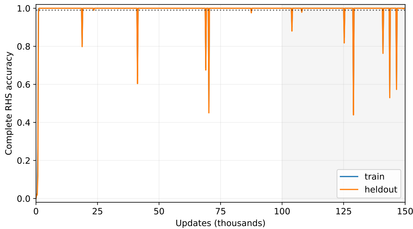
AdamW
