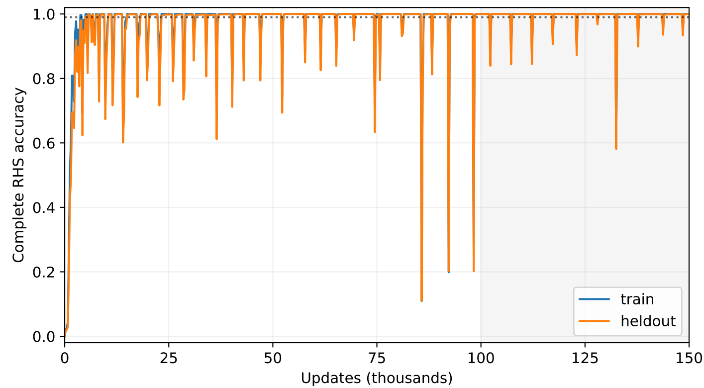
Raw AMSGradW
