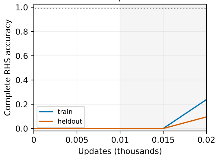
adamw-sparsemax
