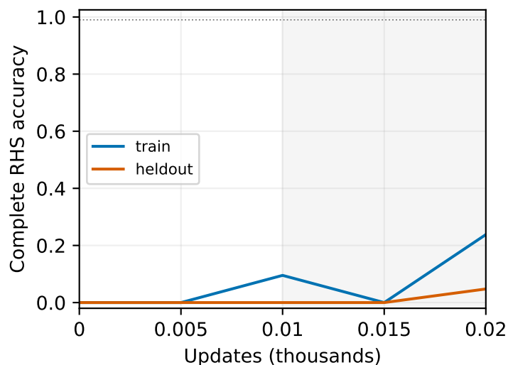
adamw-softmax
