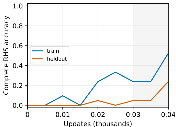
adamw-constant
