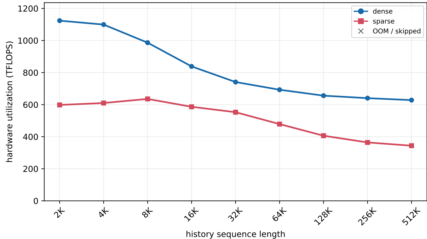
H800 MLA prefill - batch=1, new length=16K (chunked prefill)
