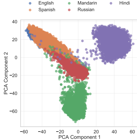
(b) Final layer language map (Llama)
