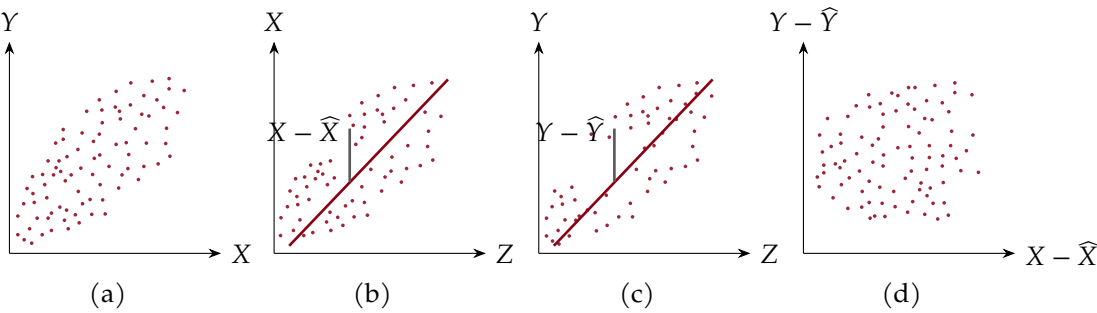
图 21.1 扣除智商的影响后, 数学成绩 Y 和语文成绩 X 之间的偏相关系数示意图 (按原书图形重绘, 点数与表 8.3 不同, 仅示意 (a)–(d) 的残差构造过程)
