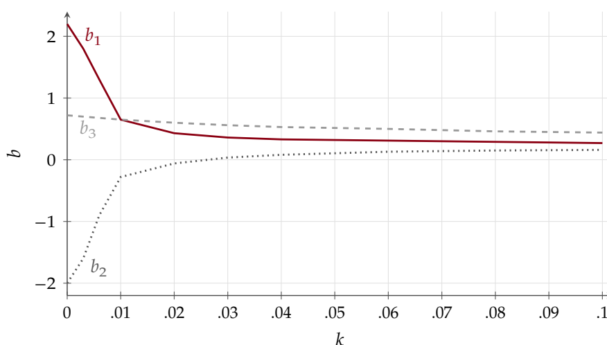
图 3.1 不同岭参数 k 时回归系数的岭迹（示意图，非由本书数据计算）
