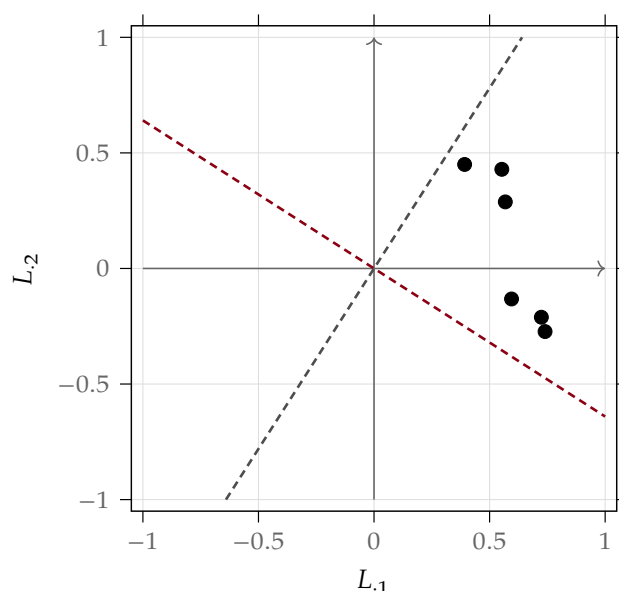
图 2.3 六门课因子负荷与正交旋转 ( 32.64386^\circ )
