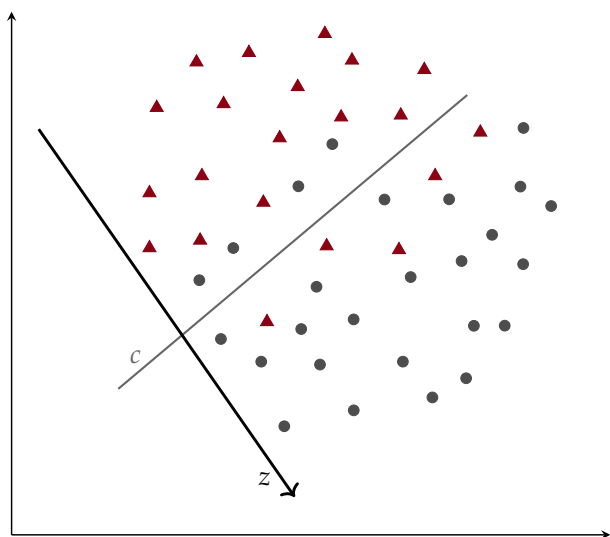
图 4.1 Fisher 判别的基本思想 (两类、两个判别指标)
