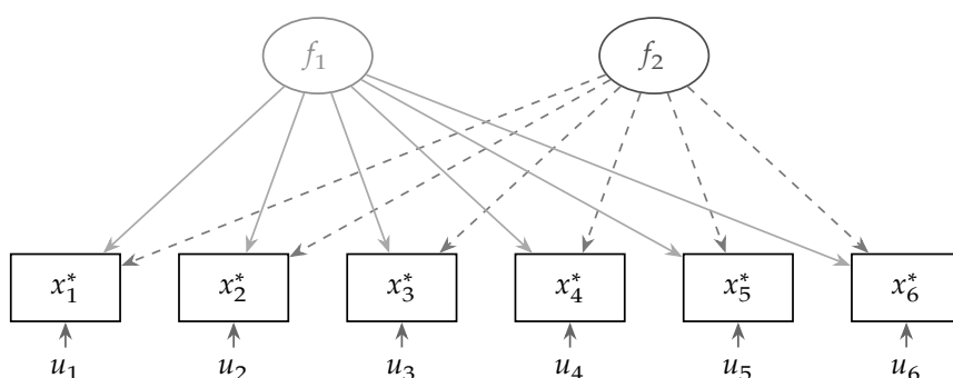
图 2.2 正交两因子模型
