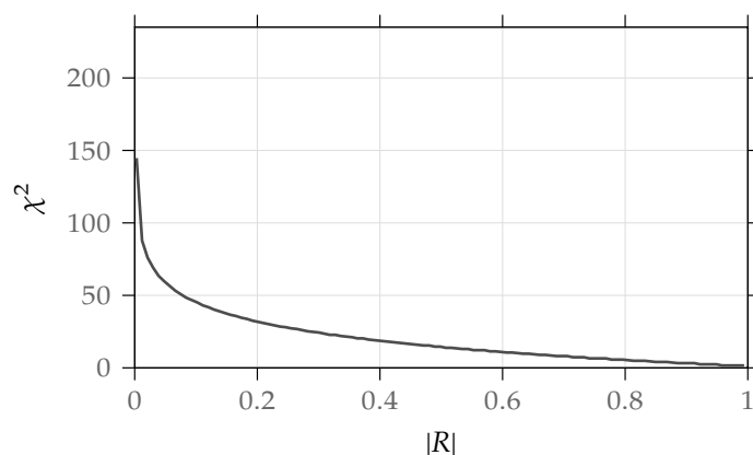
图 1.3 Bartlett 球形检验：卡方值随相关阵行列式的变化（示意图）
