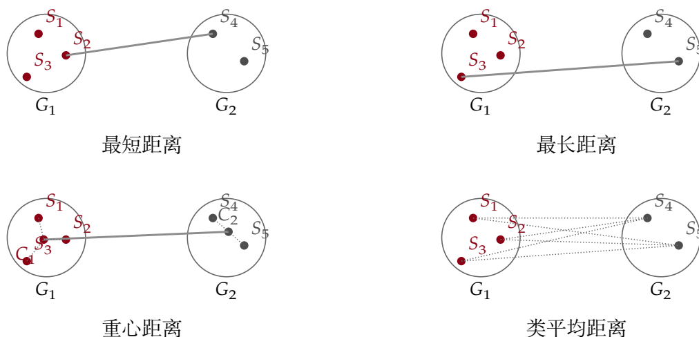
图 3.1 类间距离的四种计算方法
