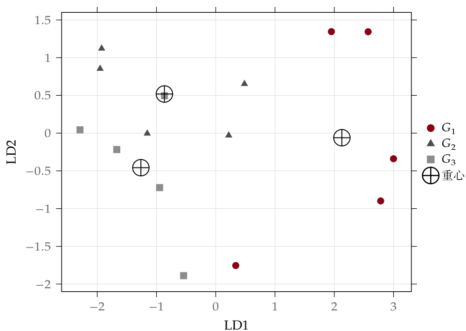
图 4.2 判别得分及各类重心
