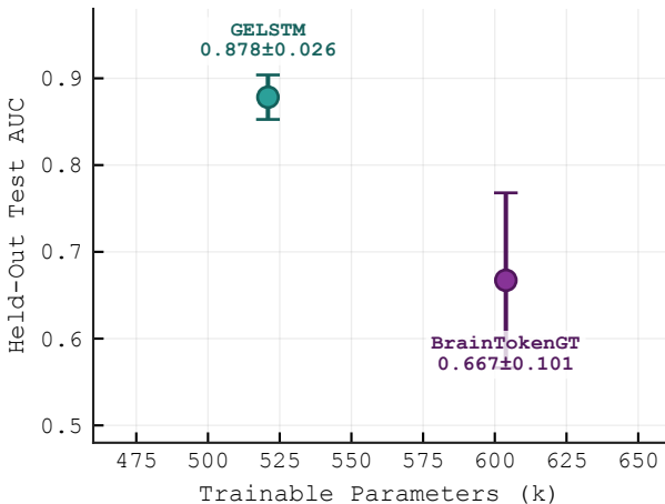
A. Parameter Efficiency Frontier
