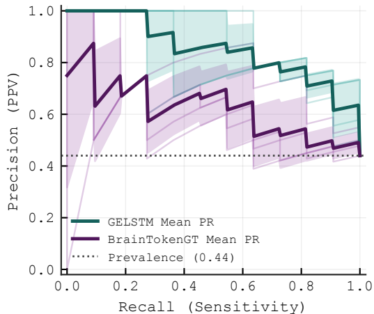
B. Precision-Recall Curves
