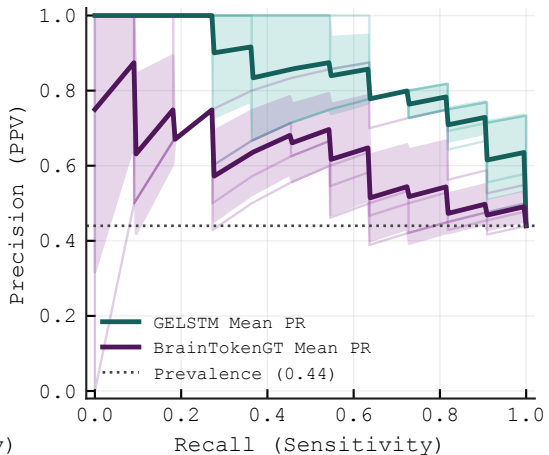
B. Precision-Recall Curves
