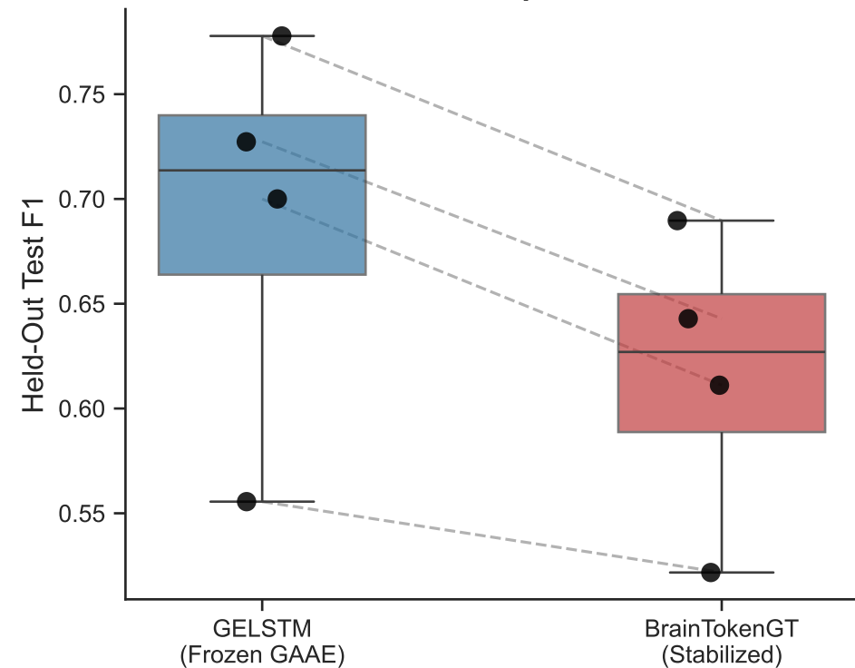
C. Held-Out Test F1 (n=4 seeds) Paired t=5.52 , p=0.0117 *
