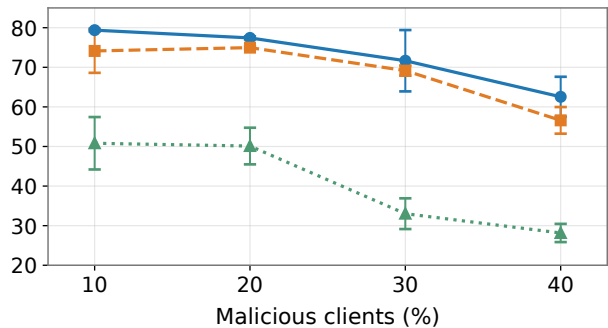
CIFAR-10 / VGG19
