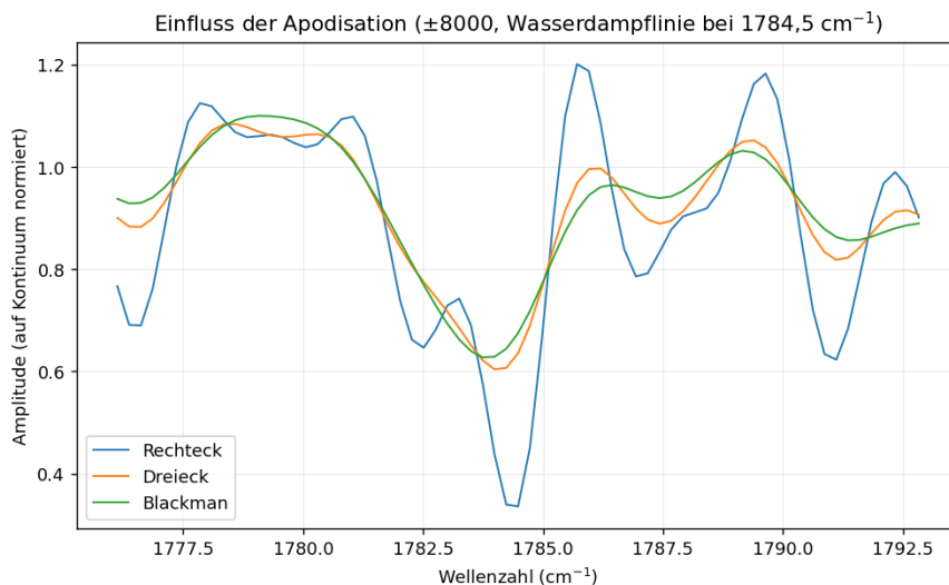
Abbildung 14: Einfluss der Apodisationsfunktion auf die isolierte Wasserdampflinie bei 1784,5 \text{ cm}^{-1} ( \pm 8000 -Messung, Zerofilling \times 4 , alle Spektren auf das lokale Kontinuum normiert). Das Rechteckfenster liefert die tiefste, schärfste Linie, zeigt aber starke Leakage-Nebenmaxima; Dreieck- und Blackman-Fenster unterdrücken diese unter Verbreiterung und Abflachung der Hauptlinie.
