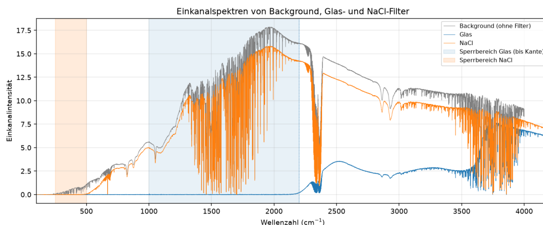
Abbildung 16: Einkanalspektren des Hintergrunds (grau) sowie des Glas- (blau) und des NaCl-Filters (orange). Farblich hinterlegt sind die Sperrbereiche. Der Glas-Sperrbereich ist bis zur tatsächlichen Sperrkante bei \approx 2200 \text{ cm}^{-1} (gepunktete Linie) markiert, bis zu der die Glaskurve flach bei null verläuft; die quantitative Auswertung erfolgt jedoch nur im rauscharmen Teilfenster (siehe Abb. 17).
