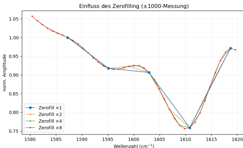
Abbildung 13: Einfluss des Zerofilling auf das Spektrum der \pm 1000 -Messung. Alle Kurven sind mit derselben Konstante normiert und laufen exakt durch die Stützstellen der unge-zerofillten Messung (blaue Punkte). Höhere Faktoren erhöhen nur die Punktdichte (Interpolation), verändern aber nicht die tatsächliche Auflösung.
