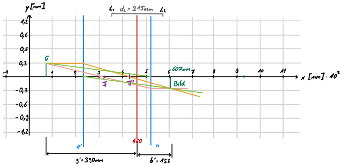
Figure 3.1: Maßstabsgetreue Skizze, mit der Entstehung des Bildes. Dabei entspricht 1 Kästchen auf der y-Achse 0.3mm und ein Kästchen auf der x-Achse 100mm
