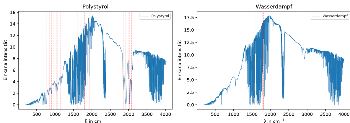
Abbildung 4: Aufgenommene Einkanalspektren von Polystyrol (links) und Wasserdampf (rechts). Die roten gepunkteten Linien markieren die zur Kalibrierung verwendeten theoretischen Wellenzahlen der Absorptionsbanden.
