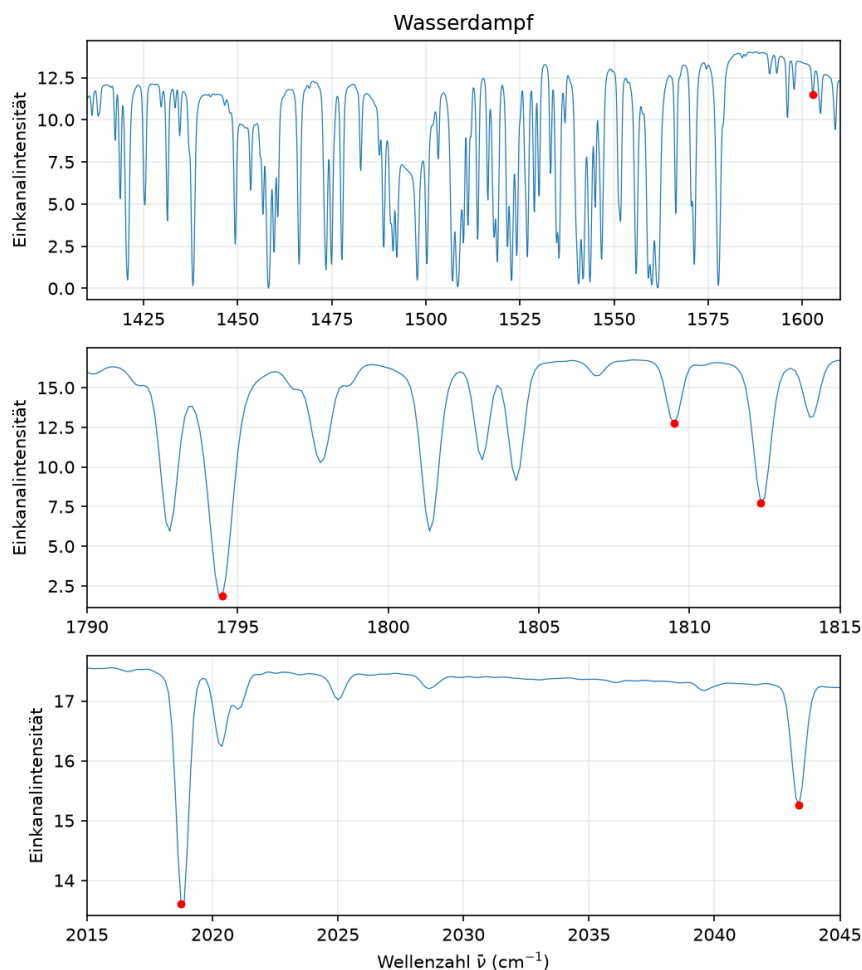
Abbildung 6: Vergrößerte Ausschnitte des Wasserdampfspektrums. Im Fenster um 1800\text{ cm}^{-1} ist erkennbar, dass die vier dicht benachbarten Referenzlinien bei der vorliegenden Auflösung nicht alle eindeutig getrennt werden können; markiert sind nur die verlässlich zuordenbaren Banden.
