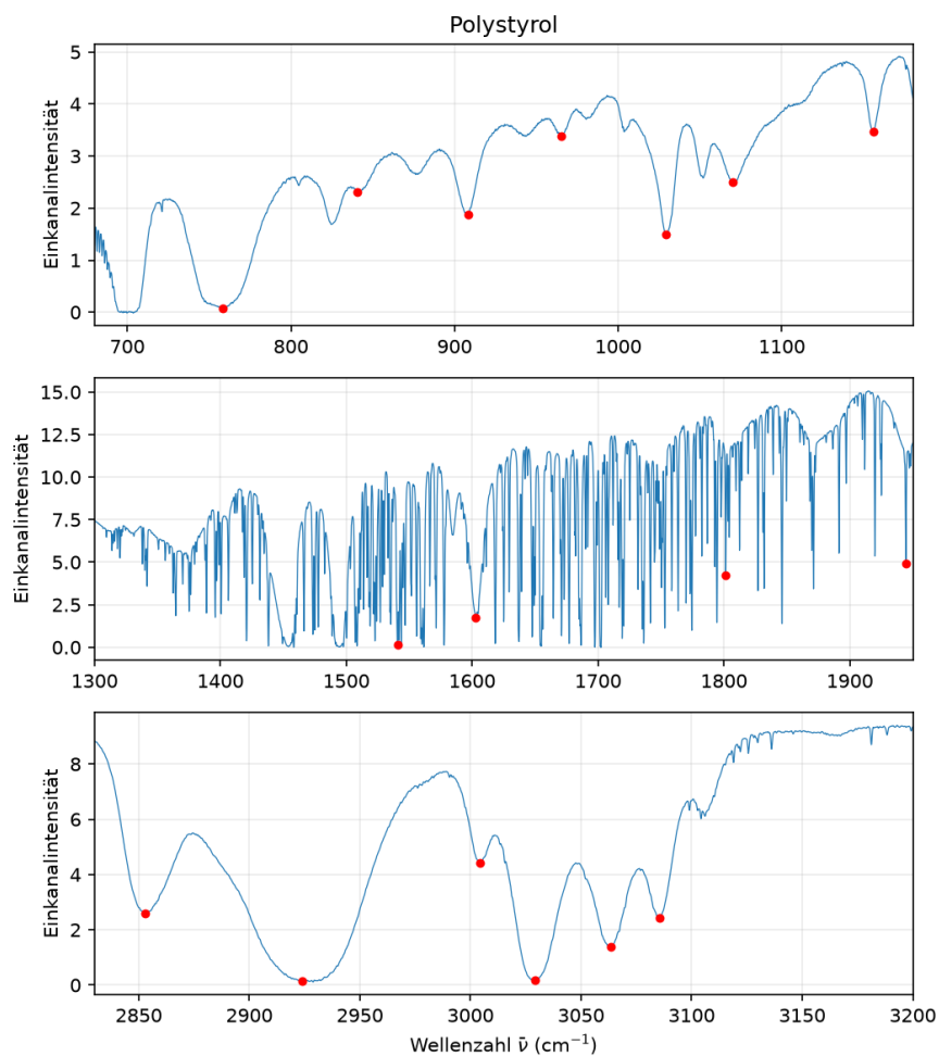
Abbildung 5: Vergrößerte Ausschnitte des Polystyrolspektrums. Rote Punkte kennzeichnen die zur Kalibrierung verwendeten Bandenminima. Die scharfen Einbrüche im mittleren Fenster stammen von Wasserdampflinien der Umgebungsluft und überlagern die breiten Polystyrolbanden.
