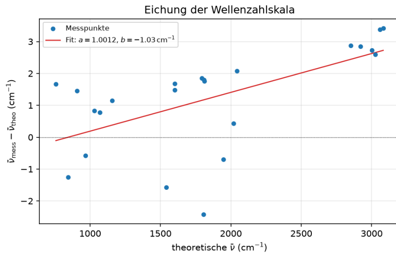
Abbildung 8: Residuendarstellung der Eichung: Differenz aus gemessener und theoretischer Wellenzahl über der theoretischen Wellenzahl. Die rote Gerade entspricht der linearen Regression \bar{\nu}_{\text{mess}} = a \bar{\nu}_{\text{theo}} + b .
