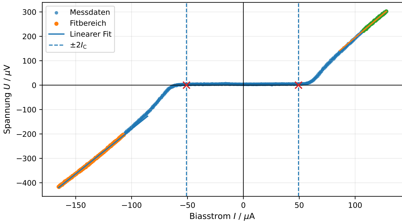
V-I-Kennlinie des DC-SQUIDs
