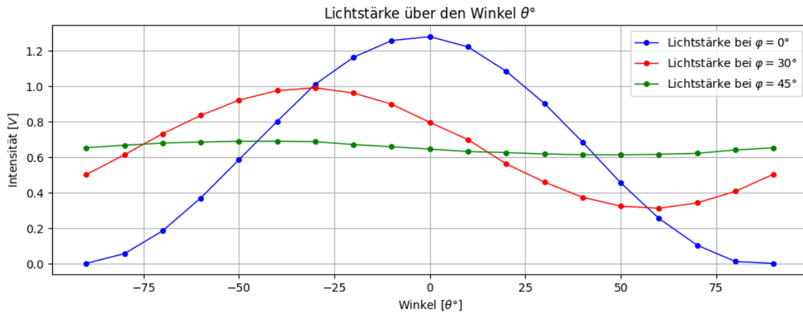
Figure 3.1: Lichtstärke in V über den Winkel \theta^\circ bei Verschiedenen \varphi^\circ vom \lambda/2 - Plättchen
