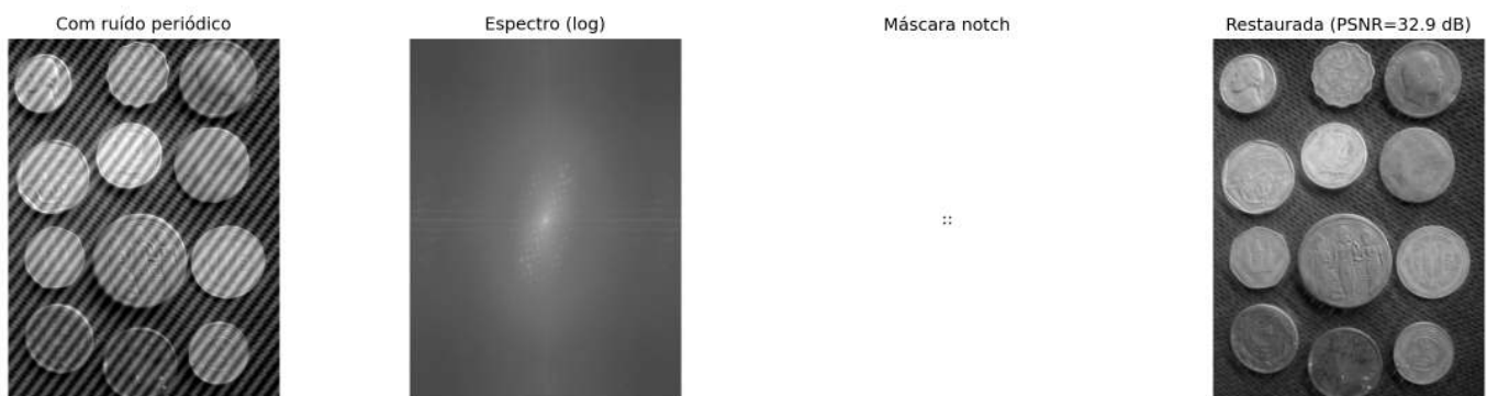
Figura 5.14: Remoção de ruído periódico via filtro notch no domínio da frequência: (a) imagem com ruído senoidal, (b) espectro mostrando os picos do ruído, (c) máscara notch centrada nos picos, (d) imagem restaurada.
