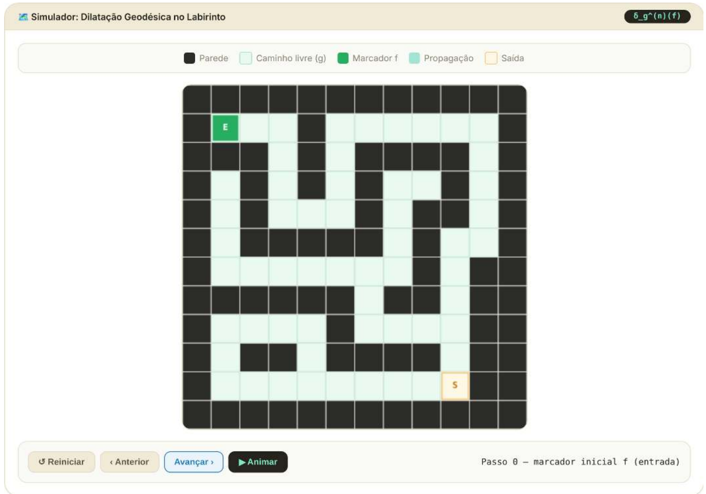
Figura 4.7: Simulador interativo de dilatação geodésica: o marcador f (verde) propaga-se passo a passo pelos caminhos livres da máscara g , sem atravessar paredes — ilustrando como \hat{g}^n(f) encontra a saída do labirinto.
