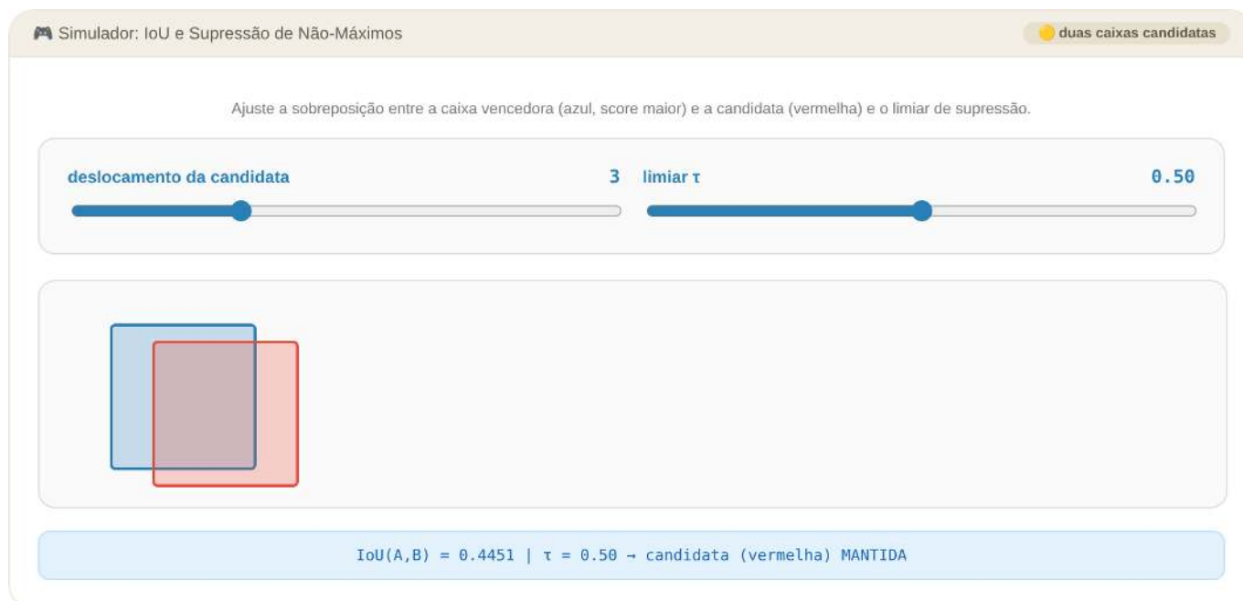
Figura 9.44: Simulador EP09_04: IoU e Supressão de Não-Máximos
