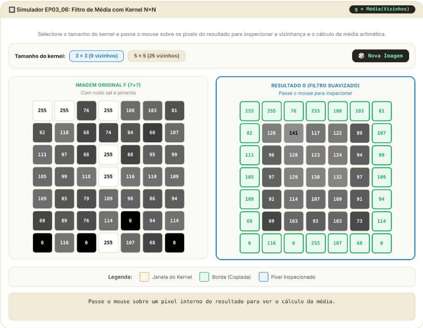
Figura 3.31: Simulador EP03_06: Filtro de Média com Kernel N×N
