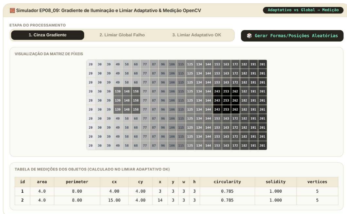
Figura 8.23: Simulador EP08 09: Gradiente de Iluminação, Limiar Adaptativo e Medição OpenCV
