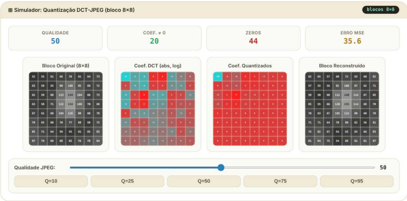
Figura 5.26: Simulador interativo de compressão DCT-JPEG: ajuste o fator de qualidade e visualize em tempo real os coeficientes zerados, o bloco reconstruído e o erro de quantização.
