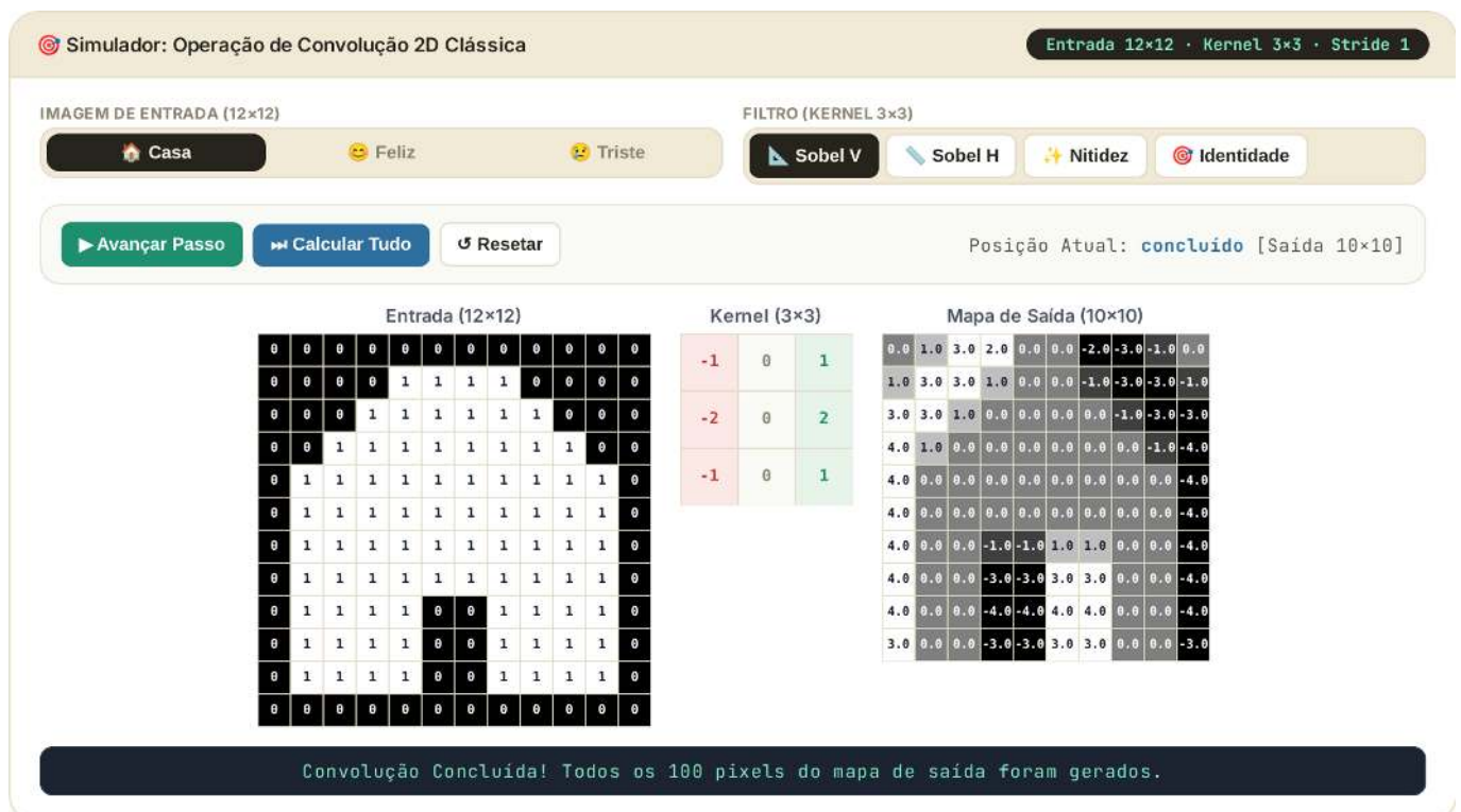
Figura 9.2: Simulador interativo de convolução 2D clássica: escolha entre as três imagens sintéticas de entrada 12×12 (casa, rosto feliz ou triste) e um filtro 3×3 (Sobel V, Sobel H, Nitidez ou Idêntidade) e avance passo a passo para observar como os produtos internos locais do campo receptivo constroem o mapa de características célula a célula.
