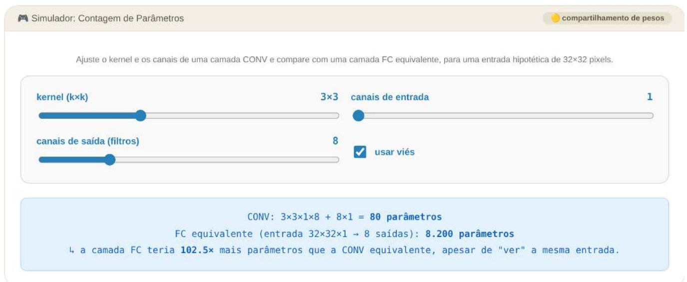
Figura 9.43: Simulador EP09_03: Contagem de Parâmetros — Convolução vs. Camada Totalmente Conectada
