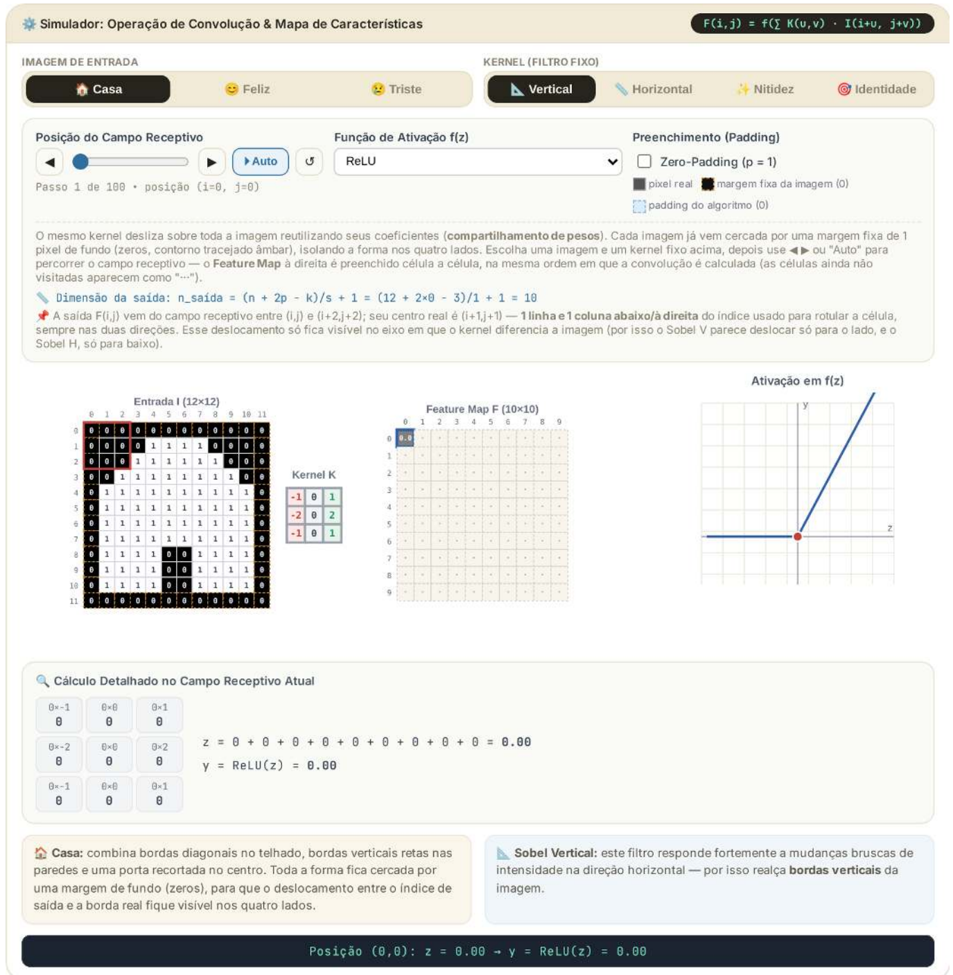
Figura 9.4: Simulador interativo da Camada Convolutiva: escolha entre três imagens de entrada 12×12 (casa, rosto feliz ou rosto triste) para observar como os mesmos kernels fixos reagem a diferentes bordas e formas. Navegue pelo campo receptivo com os botões ou reprodução automática, ajuste a função de ativação e alterne o zero-padding, acompanhando o mapa de características sendo revelado célula a célula, com o cálculo detalhado termo a termo e a fórmula da dimensão de saída em tempo real.
