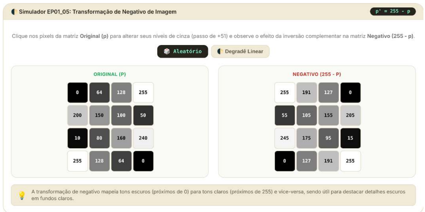
Figura 1.16: Simulador EP01_05: Transformação de Negativo de Imagem (Inversão de Intensidade)
