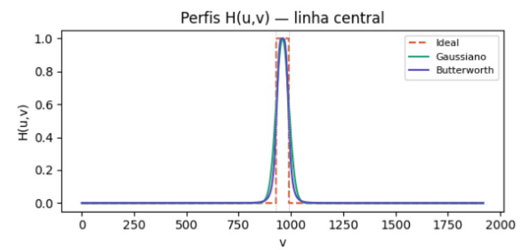
H(u,v) Profiles
