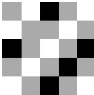
Histograma — Ecualizada
