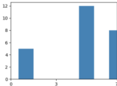
Histograma — Ecualizada
