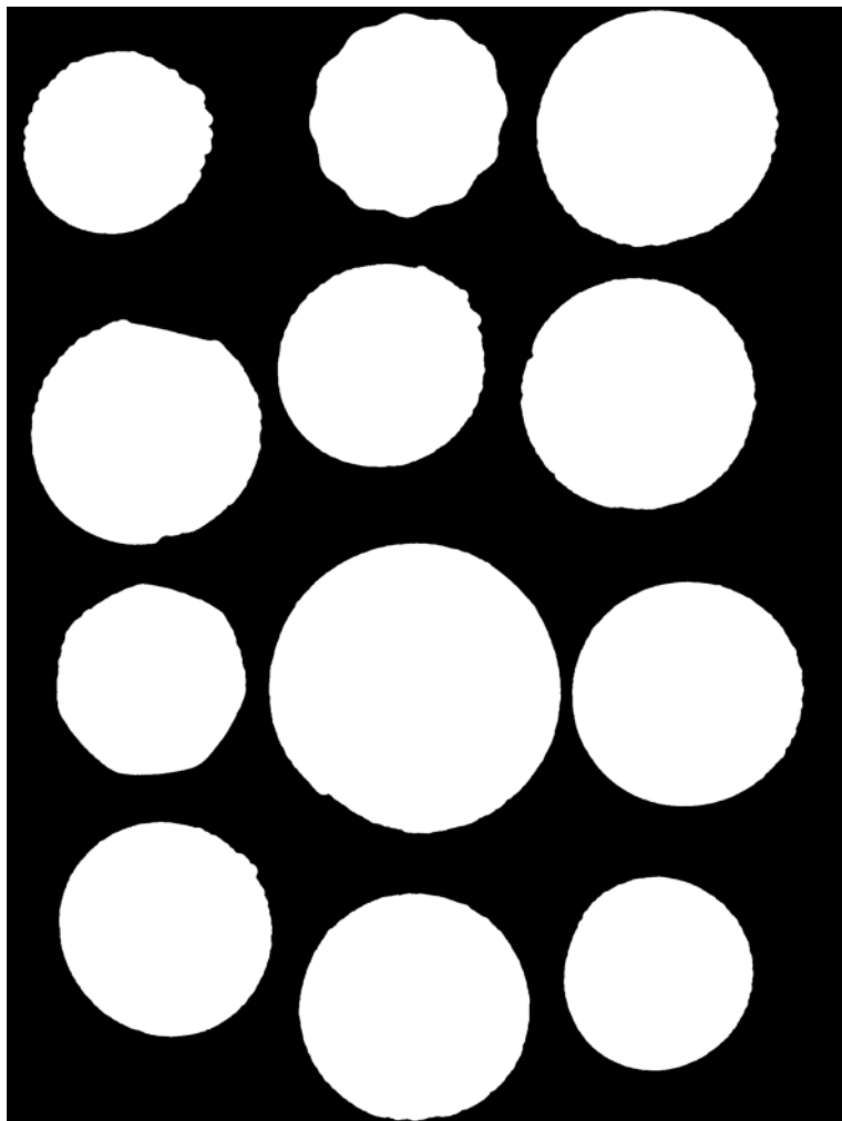
Segmentación Final
