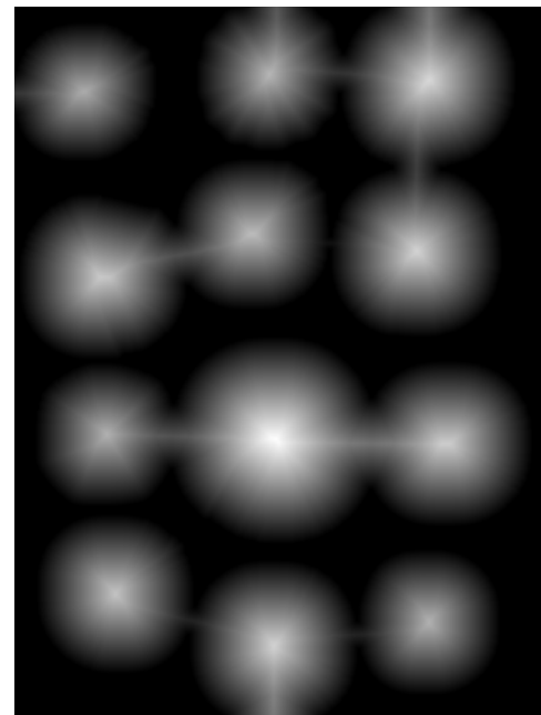
Anotado
