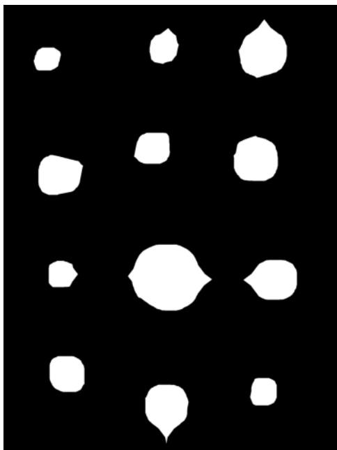
Marcadores
