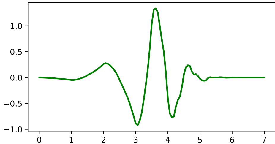
Ondaleta Daubechies 4 ( \psi )
