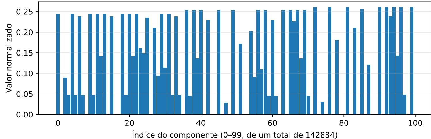
Primeiros componentes do vetor HOG
