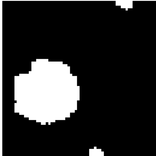
Prédiction classique
