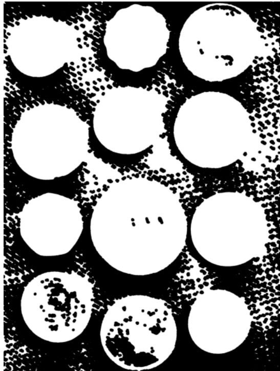
Fechamento ( A \circ B )
