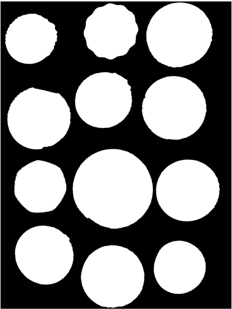
Segmentación Final
