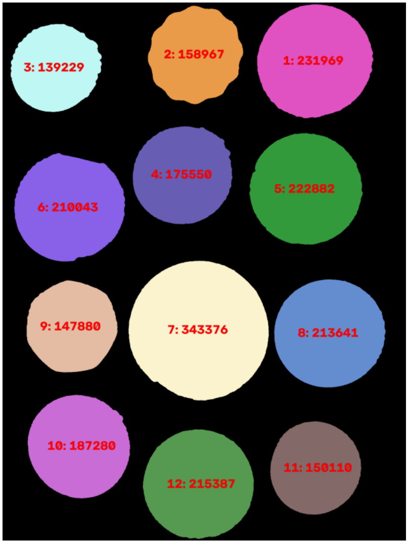
Áreas Anotadas
