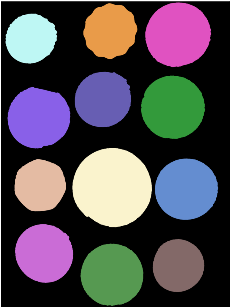
Componentes Conexos
