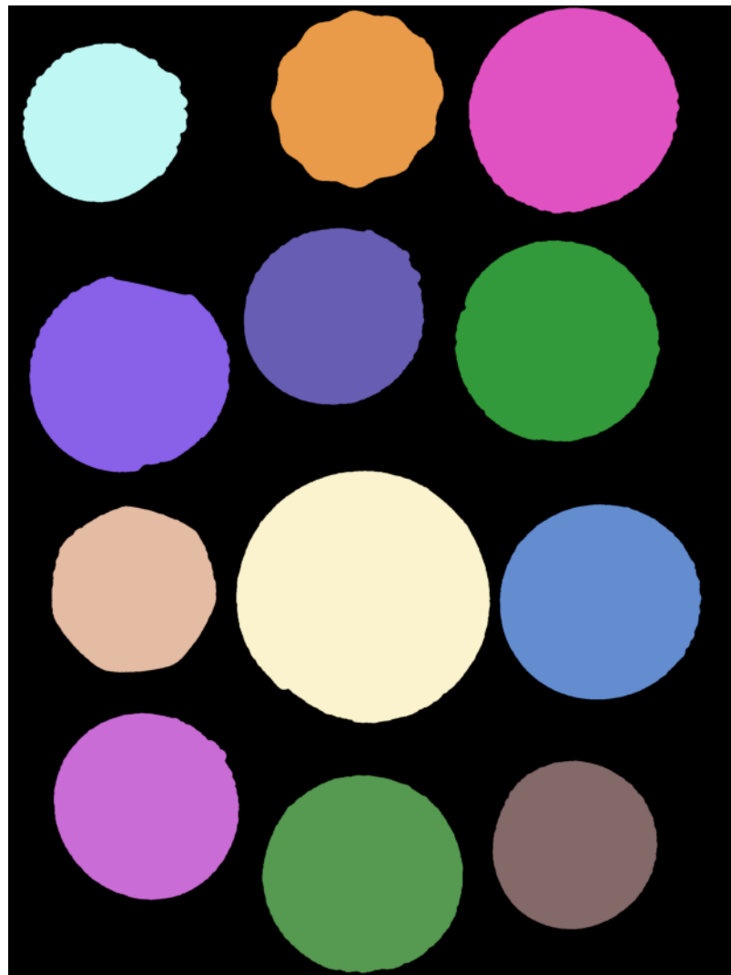
Composantes Connexes
