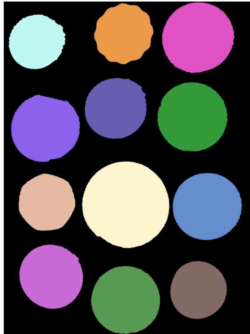
Componenti Connessi
