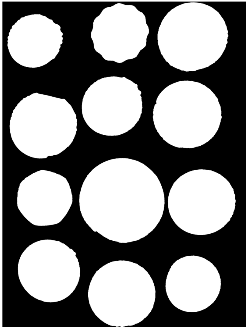
Segmentazione Finale
