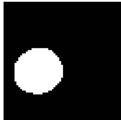
Amostra 2: U-Net
