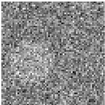
Amostra 2: Imagem
