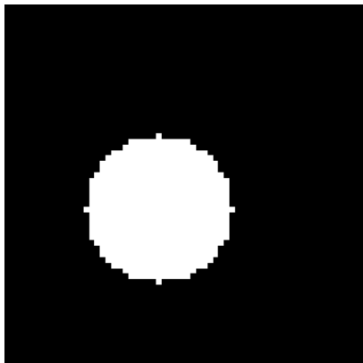
Amostra 3: Referência
