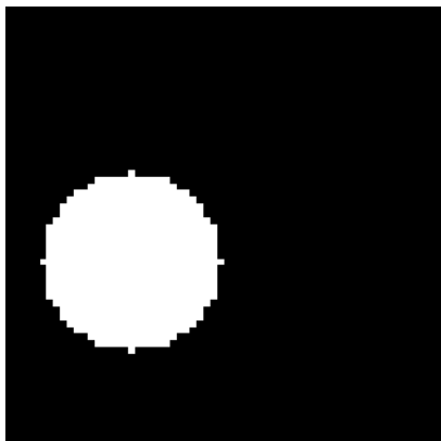
Amostra 2: Referência
