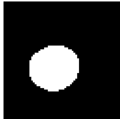
Amostra 3: U-Net
