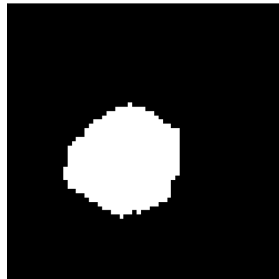
Amostra 3: Clássico
