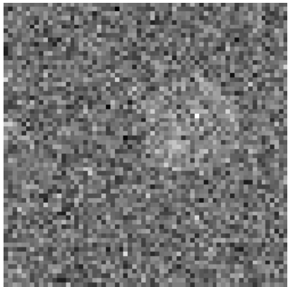
Amostra 3: Imagem
