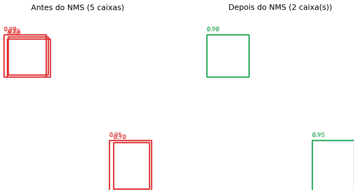
Figura 8.10: Efeito da Supressão de Não-Máximos (NMS): múltiplas detecções redundantes (esquerda) são reduzidas a uma detecção por objeto (direita).
