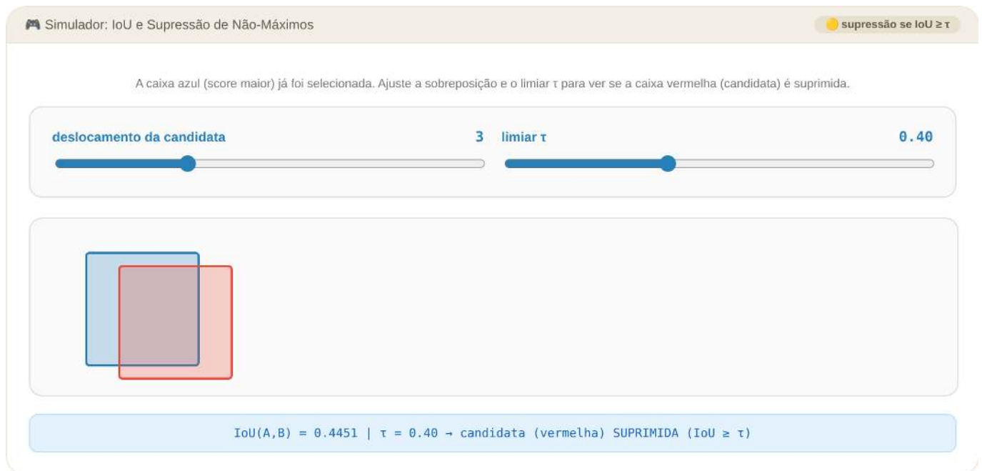
Figura 8.18: Simulador: IoU e Supressão de Não-Máximos
