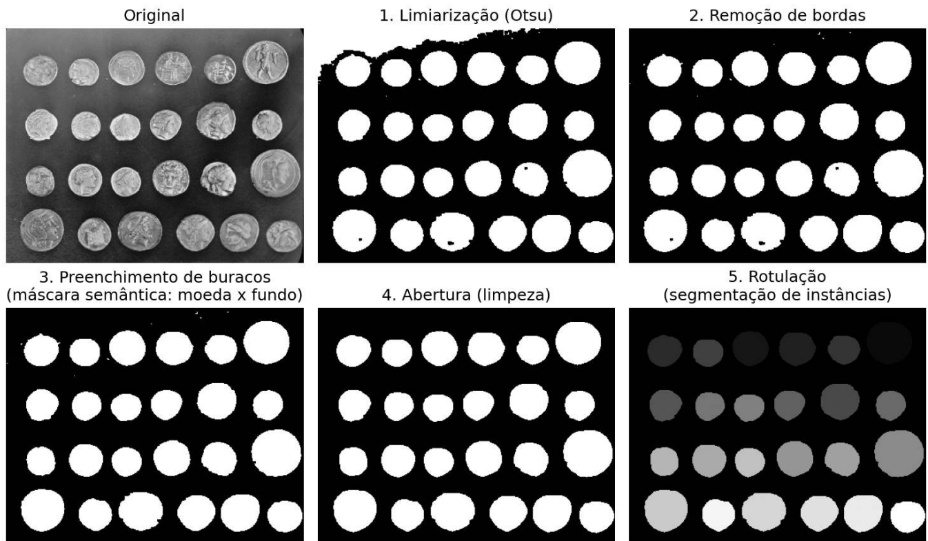
Figura 8.12: Segmentação clássica (não baseada em aprendizado profundo): máscara semântica (moeda x fundo) via limiarização de Otsu, e segmentação de instâncias via rotulação de componentes conectados.
