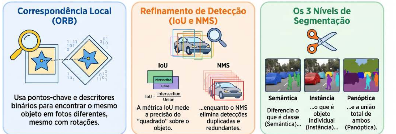
Figura 8.1: Visão geral dos principais conceitos abordados neste capítulo, incluindo correspondência de características, detecção de objetos, segmentação de imagens e suas relações com abordagens modernas baseadas em Deep Learning . Fonte: elaborado com auxílio do Gemini Notebook (Google, 2025).
