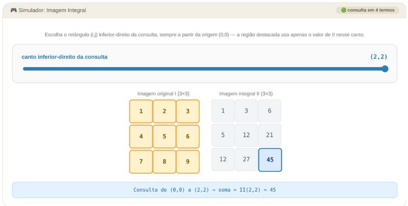
Figura 8.17: Simulador: Imagem Integral e Consulta Retangular em O(1)
