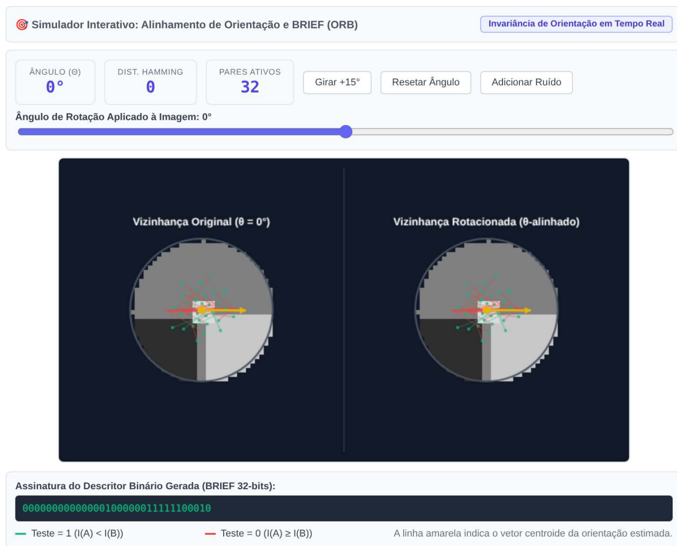
Figura 8.3: Simulador interativo do descritor ORB: explore a lógica de rotação e construção do descritor binário. Altere a rotação para observar como o padrão de amostragem de testes binários do BRIEF (linhas verdes e vermelhas) se orienta dinamicamente para garantir a invariância angular.
