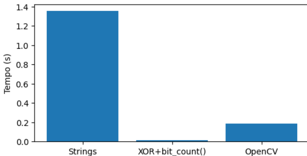
Figura 8.2: Comparação do desempenho de diferentes implementações da distância de Hamming.
