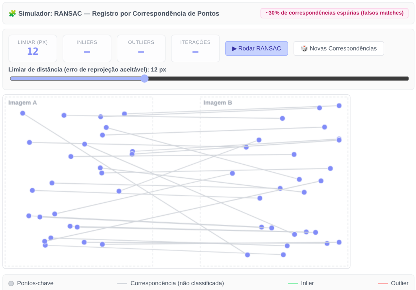
Figura 8.7: Simulador interativo do RANSAC aplicado ao registro de imagens: pontos-chave de duas imagens são casados por um descritor, algumas correspondências são espúrias ( outliers ), e o RANSAC estima a transformação de similaridade que alinha a maioria delas.
