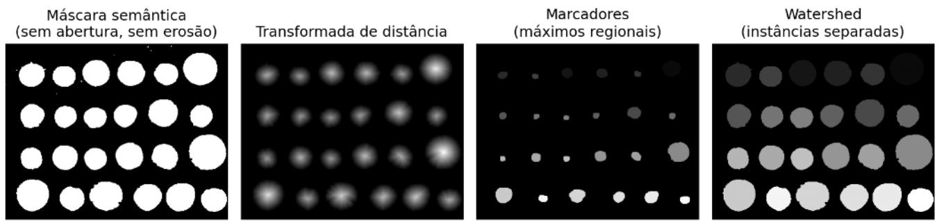
Figura 8.13: Separação de moedas que se tocam via transformada de distância + watershed , sem erosão do contorno das moedas.
