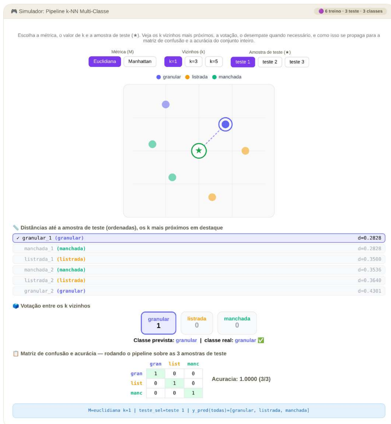
Figura 7.26: Simulador: Pipeline k-NN Multi-Classe (votacao, desempate e matriz de confusao)
