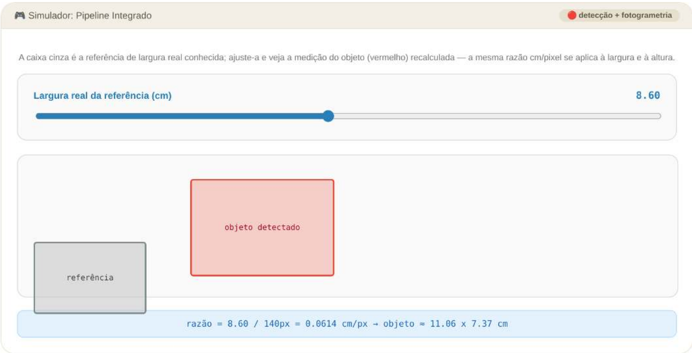
Figura 9.42: Simulador: Pipeline Integrado — NMS + Medição por Referência de Escala
