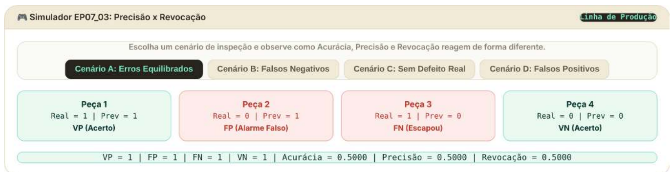
Figura 7.23: Simulador: Precisão x Revocação
