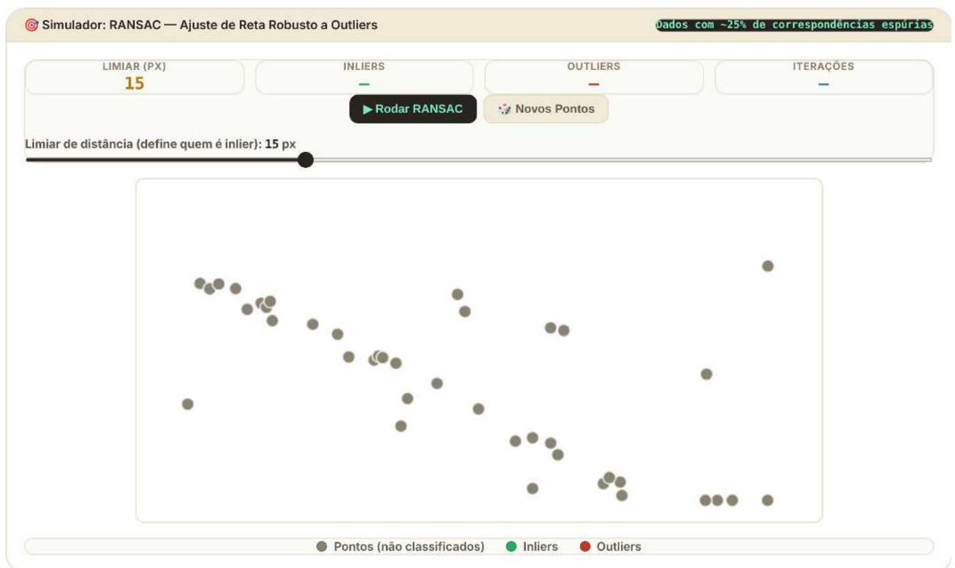
Figura 8.6: Simulador interativo do algoritmo RANSAC: ajuste o limiar de distância e execute o algoritmo para observar a separação entre inliers e outliers .
