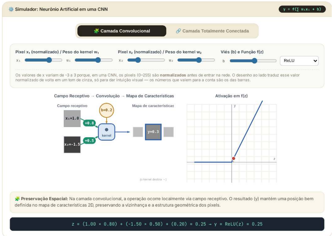
Figura 9.3: Simulador interativo do Neurônio Artificial em contexto de CNN: alterne entre um neurônio de camada convolutiva (onde x_i são intensidades de pixel em um campo receptivo e w_i são pesos do kernel ) e um neurônio de camada totalmente conectada, ajustando entradas, pesos, viés e função de ativação para visualizar o cálculo de z e da saída y em tempo real.
