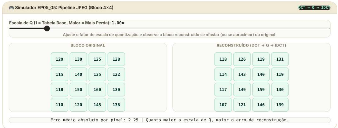
Figura 5.36: Simulador: Pipeline JPEG completo em bloco
