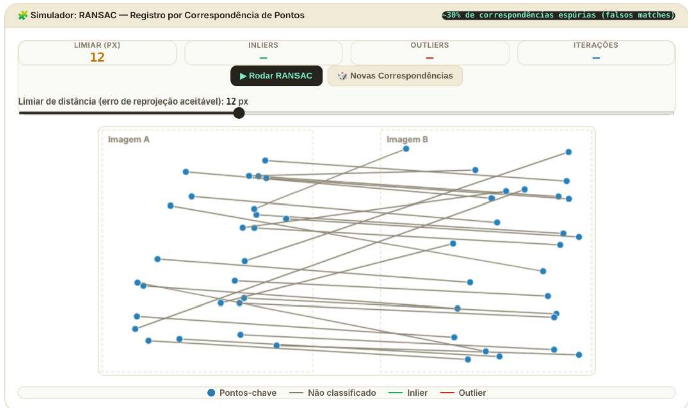
Figura 8.7: Simulador interativo do RANSAC aplicado ao registro de imagens: pontos-chave de duas imagens são casados por um descritor, algumas correspondências são espúrias ( outliers ), e o RANSAC estima a transformação de similaridade que alinha a maioria delas.
