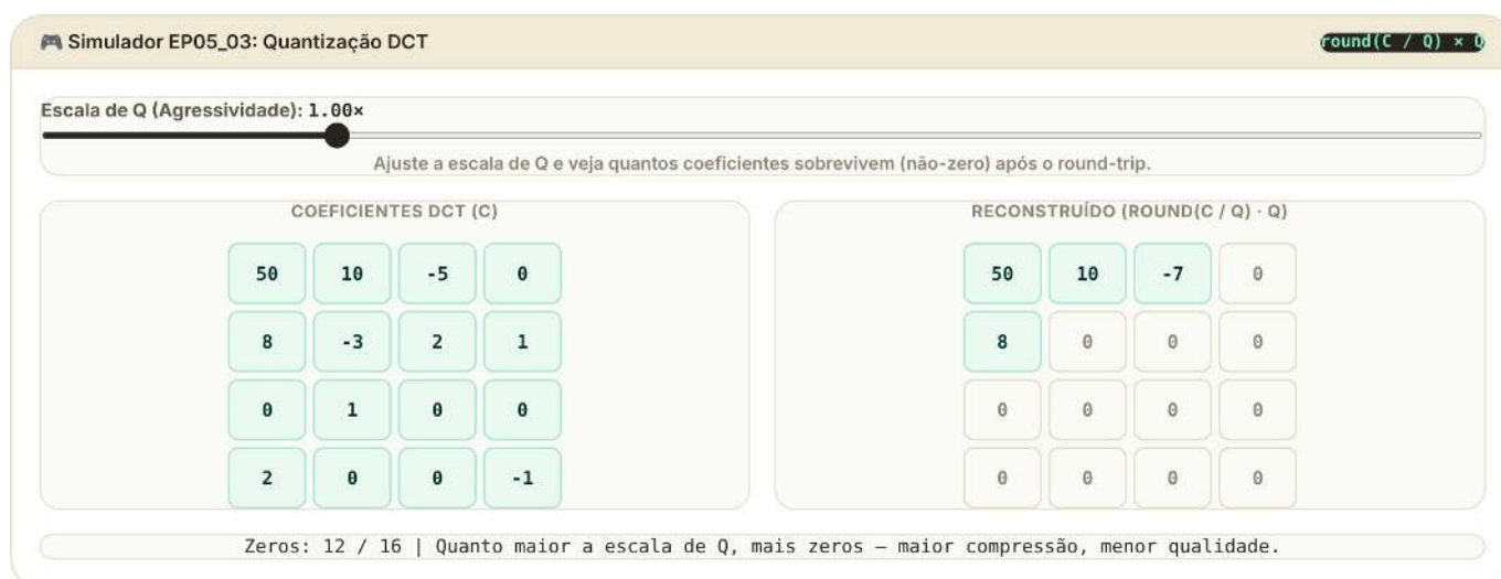
Figura 5.34: Simulador: Quantização DCT (round-trip)
