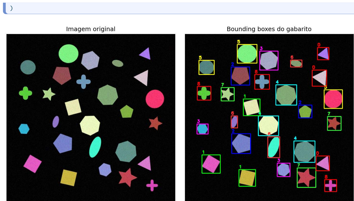
Figura 8.26: Simulador: Imagem utilizada no EP08_12. À esquerda, a imagem original. À direita, a imagem com as bounding boxes do arquivo de gabarito.
