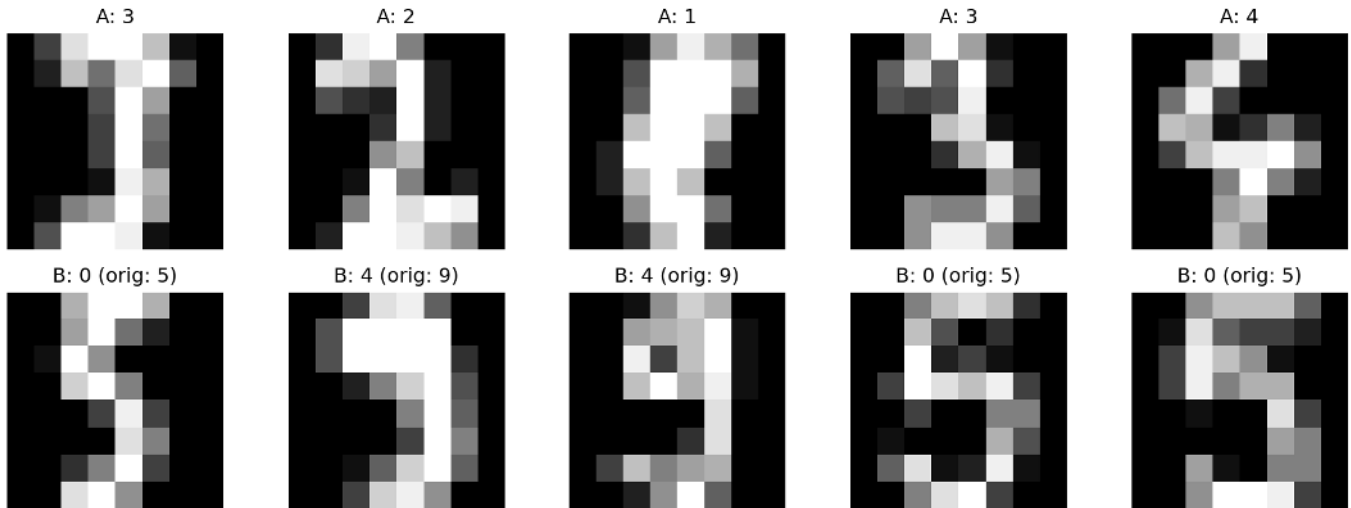
Figura 9.20: Amostras dos conjuntos de treinamento após pré-processamento e adequação dimensional aos tensores PyTorch: Domínio A (dígitos 0 a 4, tarefa de origem) e Domínio B (dígitos 5 a 9 reindexados para 0 a 4, tarefa de destino).
