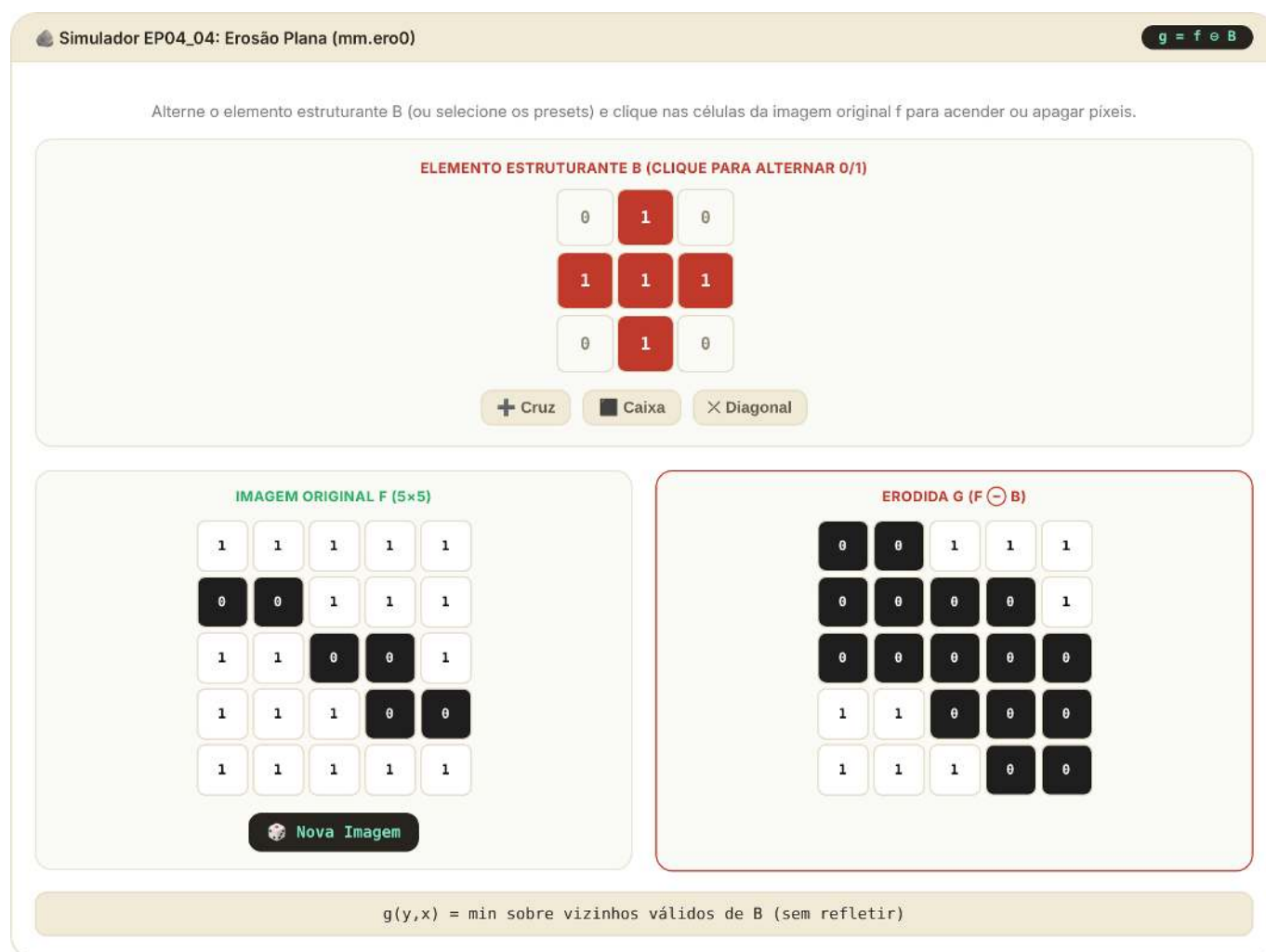
Figura 4.33: Simulador EP04_04: Erosão Binária Plana ( g = f \ominus B )
