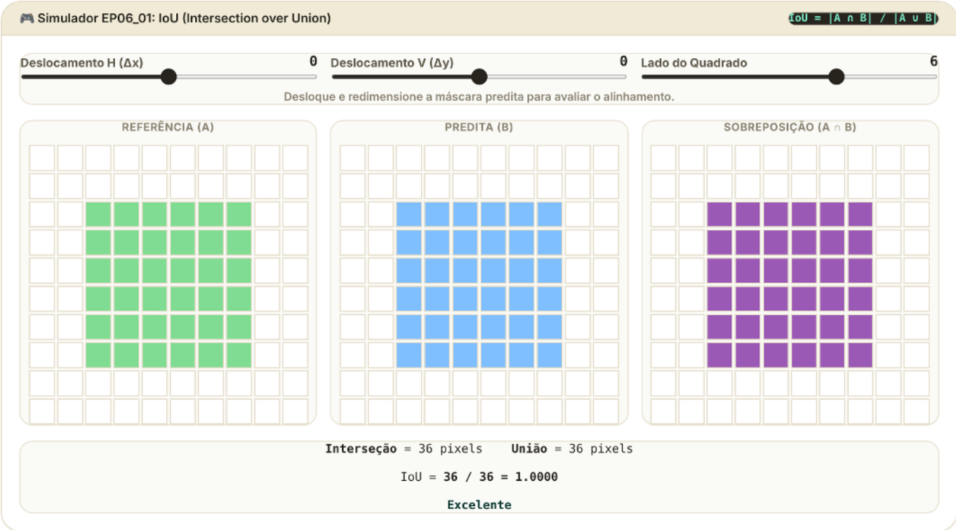
Figura 6.21: Simulador: IoU entre máscara de referência e máscara predita
