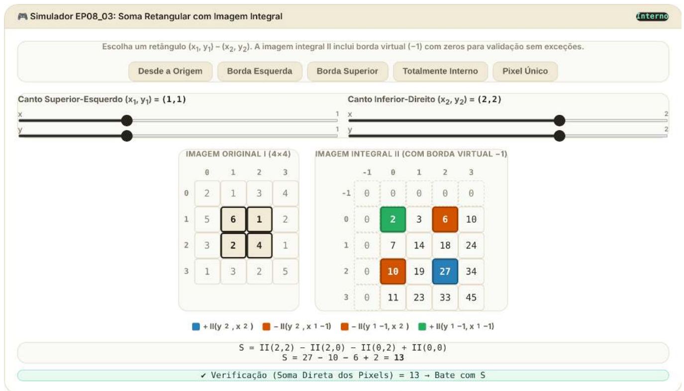
Figura 8.17: Simulador: Soma Retangular em O(1) — Múltiplas Situações de Borda
