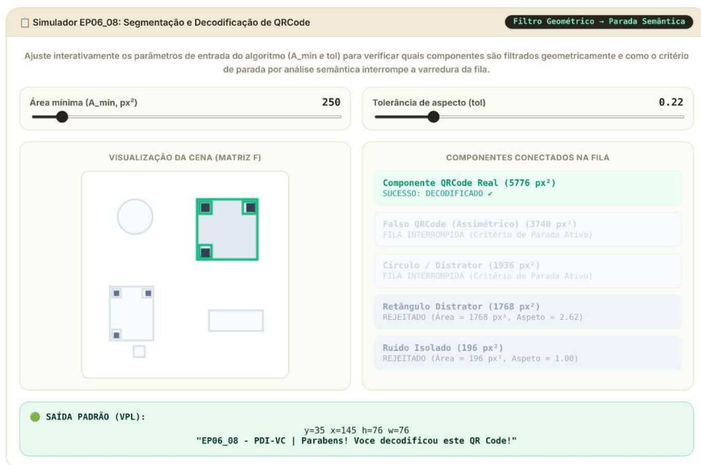
Figura 6.28: Simulador: Segmentação Geométrica + Verificação por Decodificação de QRCode
