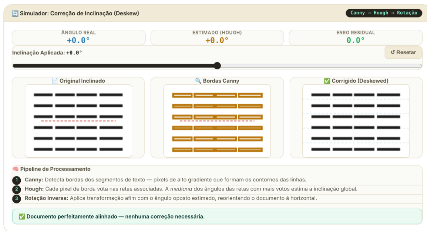
Figura 6.6: Simulador interativo de correção de inclinação ( deskew ): mova o slider para inclinar o documento e observe as três etapas do pipeline — imagem inclinada, bordas Canny e resultado corrigido.
