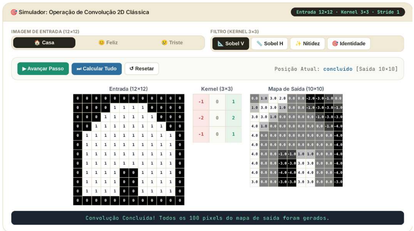
Figura 9.2: Simulador interativo de convolução 2D clássica: escolha entre as três imagens sintéticas de entrada 12x12 (casa, rosto feliz ou triste) e um filtro 3x3 (Sobel V, Sobel H, Nitidez ou Identidade) e avance passo a passo para observar como os produtos internos locais do campo receptivo constroem o mapa de características célula a célula.
