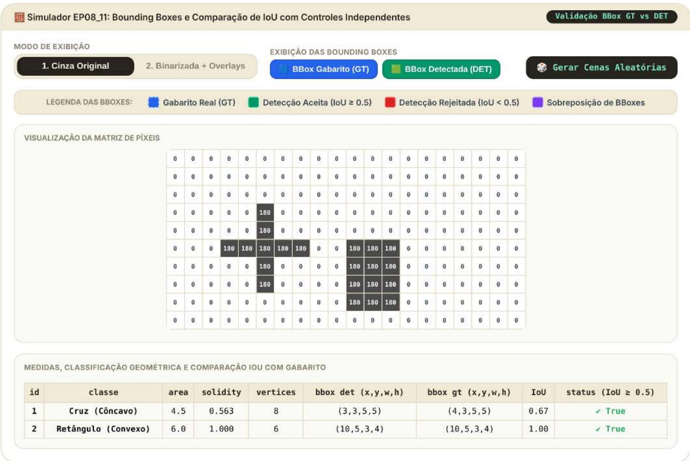
Figura 8.25: Simulador: Classificação Geométrica com Controles Independentes de Overlays BBox (GT e DET)
