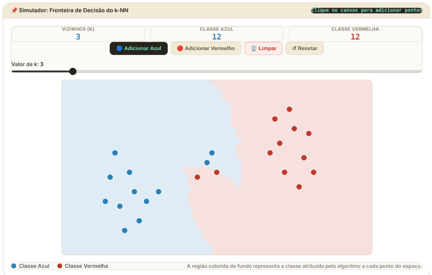
Figura 7.12: Simulador interativo da fronteira de decisão do k-NN: adicione pontos de treinamento e ajuste o valor de k para observar o efeito sobre a região de decisão.
