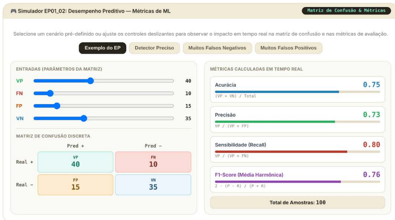
Figura 1.13: Simulador EP01_02: Desempenho Preditivo — Métricas de ML
