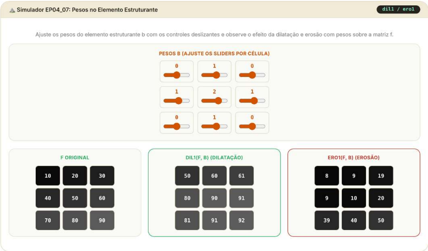
Figura 4.36: Simulador EP04_07: Dilatação e Erosão com Pesos (mm.dill1 / mm.erol)
