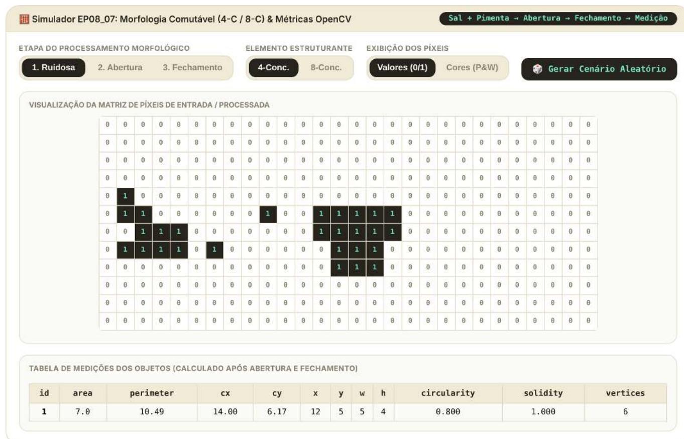
Figura 8.21: Simulador: Morfologia com Conectividade Configurável e Medição
