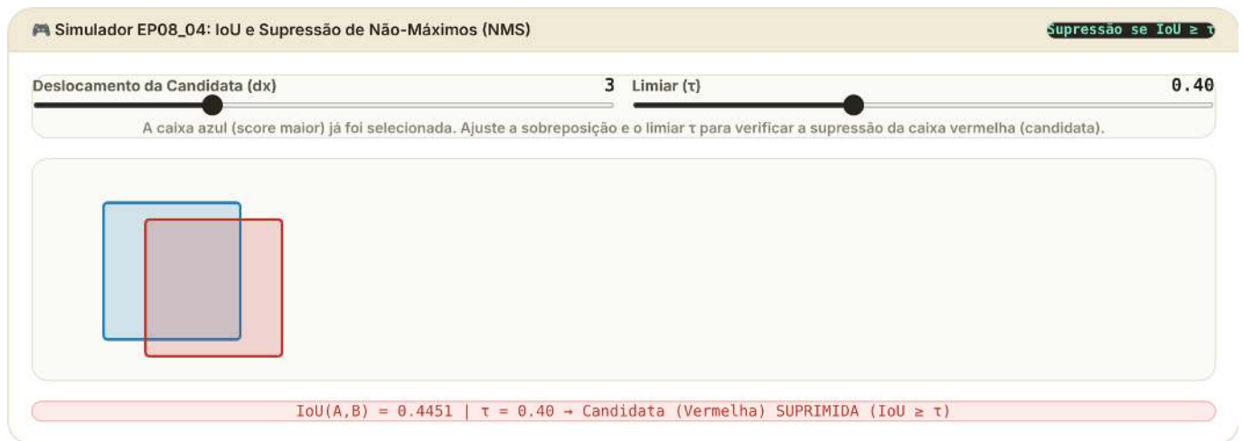
Figura 8.18: Simulador: IoU e Supressão de Não-Máximos
