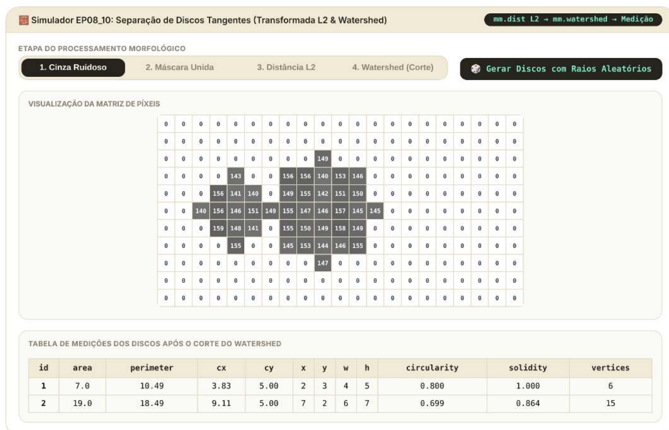
Figura 8.24: Simulador: Separação de Discos Tangentes via Transformada de Distância L2 e Watershed
