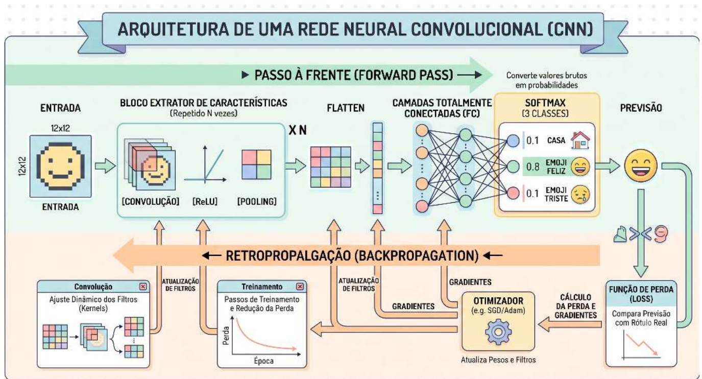
Figura 9.10: Arquitetura simplificada de uma CNN para classificação de imagens, destacando o forward pass e as etapas de treinamento por meio da função de perda, da retropropagação e do algoritmo de otimização.
