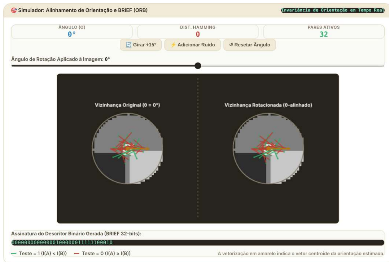
Figura 8.3: Simulador interativo do descritor ORB: explore a lógica de rotação e construção do descritor binário. Altere a rotação para observar como o padrão de amostragem de testes binários do BRIEF (linhas verdes e vermelhas) se orienta dinamicamente para garantir a invariância angular.
