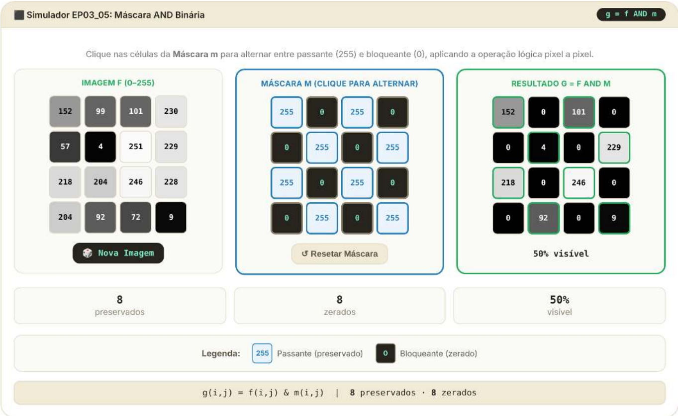
Figura 3.30: Simulador: Aplicação de Máscara AND Binária
