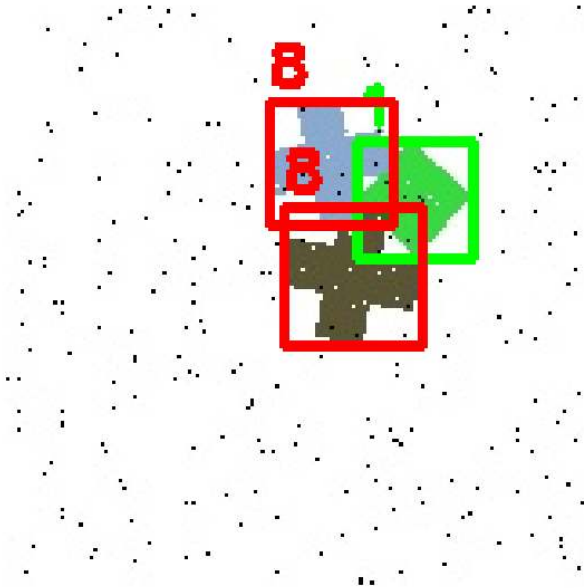
Figura 9.29: Comparativo entre a imagem ruidosa original do dataset sintético e a versão restaurada via Filtro de Mediana com as anotações YOLO sobrepostas.
