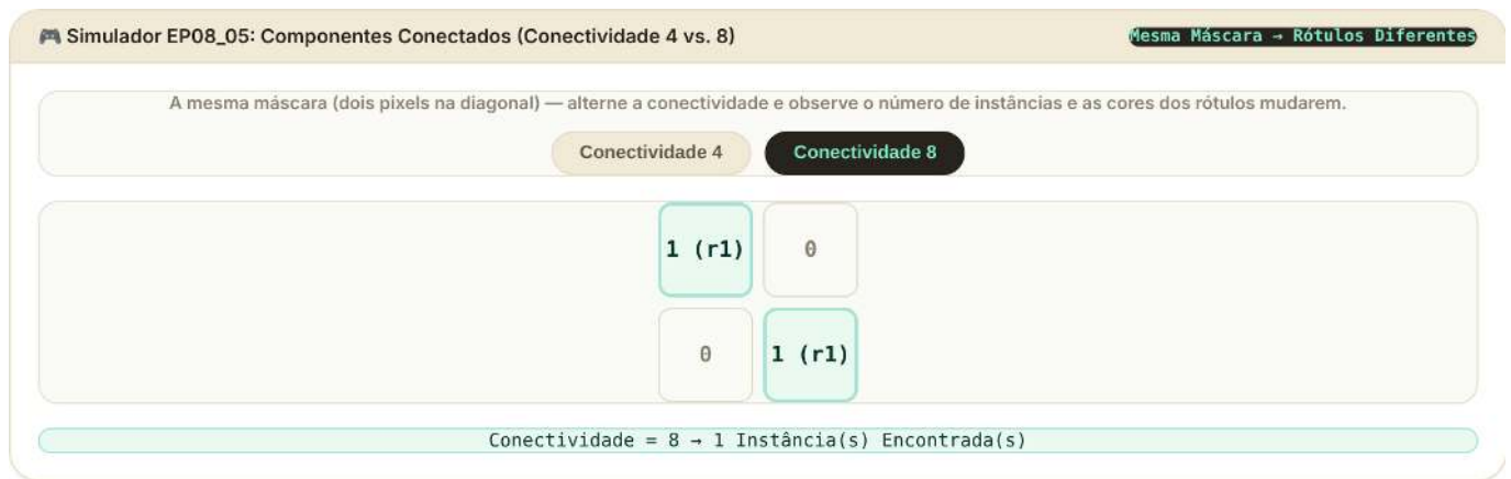
Figura 8.19: Simulador: Rotulação de Componentes Conectados — Conectividade 4 vs. 8
