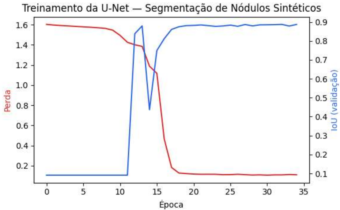
Figura 9.33: Evolução do treinamento da U-Net compacta: redução da perda e elevação do índice IoU médio no conjunto de validação ao longo de 35 épocas.
