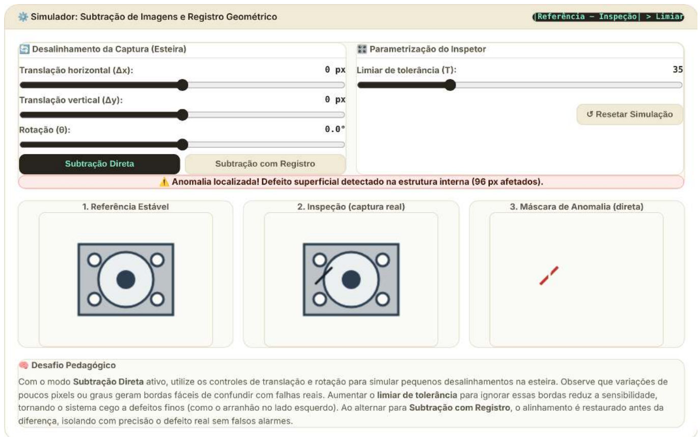
Figura 6.19: Simulador interativo de inspeção industrial por subtração de imagens: controle as distorções geométricas de desalinhamento (registro) e o limiar de detecção para observar o impacto nos falsos positivos.
