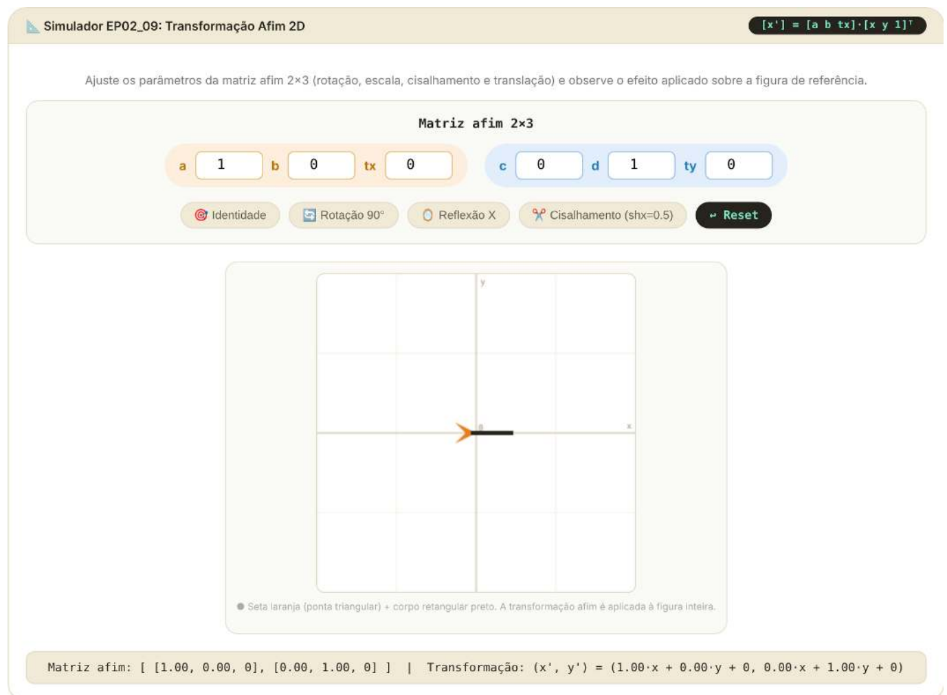
Figura 2.20: Simulador EP02_09: Transformação Afim 2D (Matriz 2×3)
