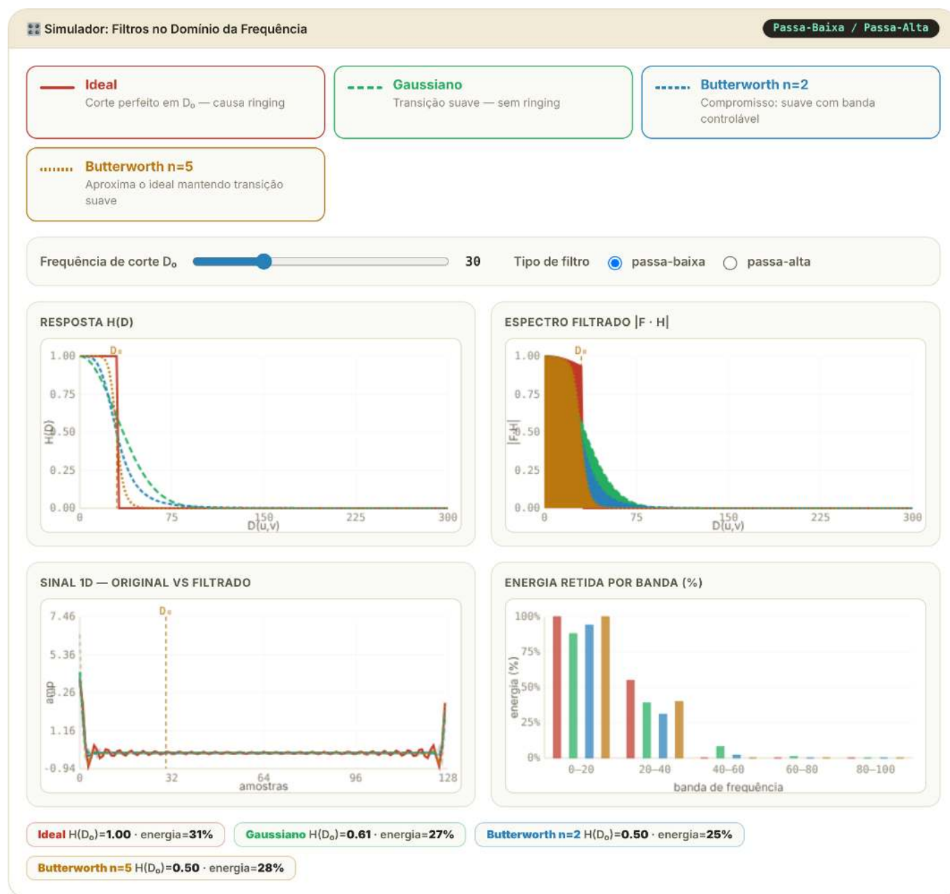
Figura 5.12: Simulador interativo de filtros no domínio da frequência.
