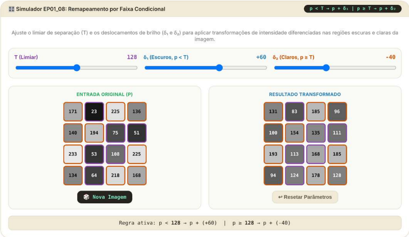
Figura 1.19: Simulador EP01_08: Remapeamento por Faixa Condicional (Brilho e Contraste por Limiar)
