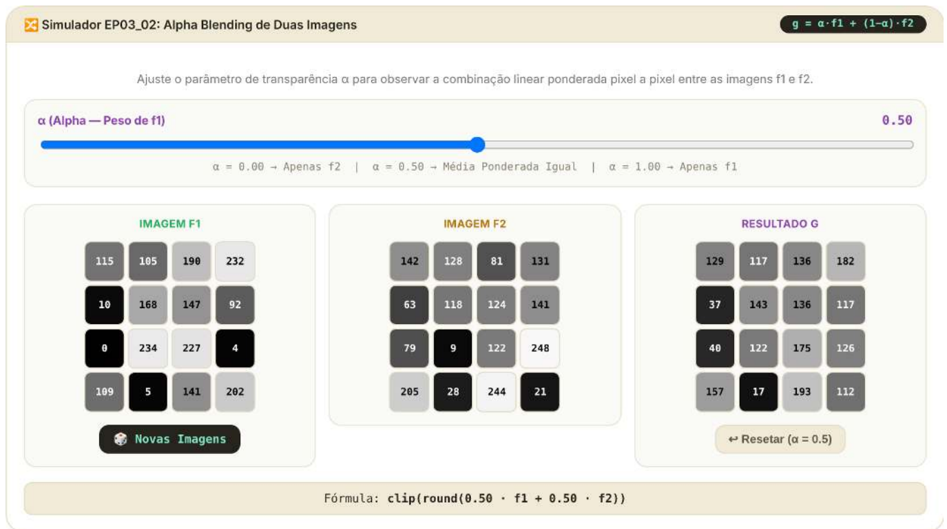
Figura 3.27: Simulador EP03_02: Alpha Blending de Duas Imagens ( g = \alpha \cdot f1 + (1-\alpha) \cdot f2 )
