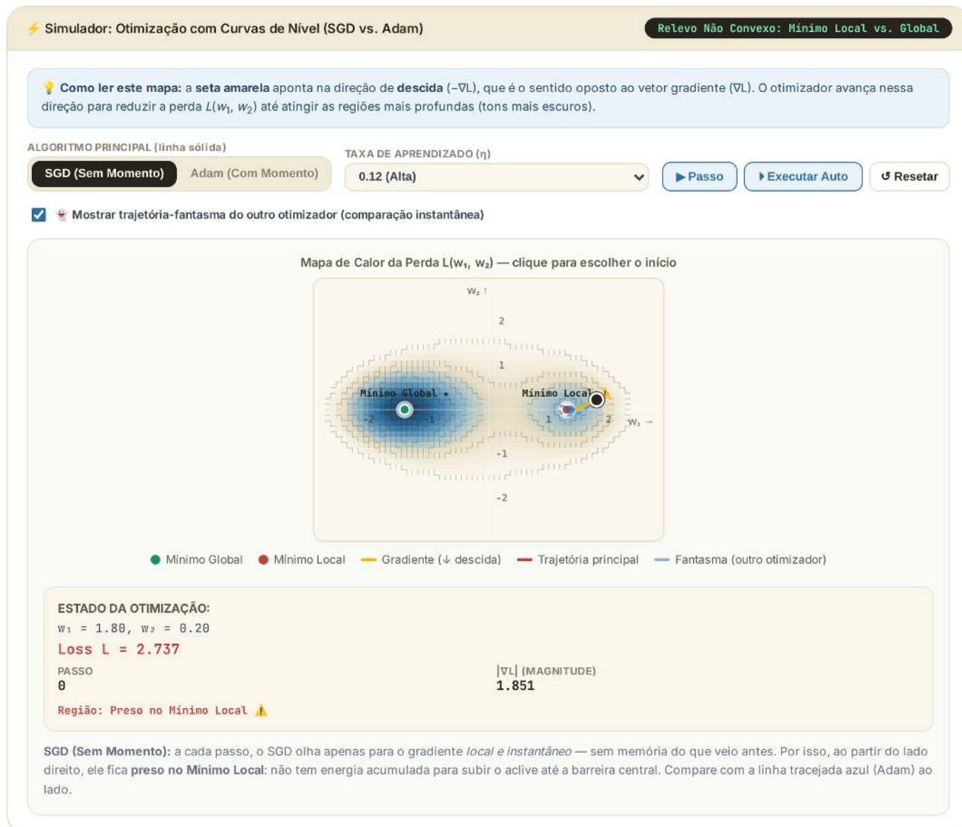
Figura 9.9: Simulador interativo dos Algoritmos de Otimização: compare a trajetória do SGD e do Adam sobre uma superfície de perda não convexa com mapa de calor e curvas de nível. A linha sólida mostra o otimizador selecionado avançando passo a passo; a linha tracejada mostra, para comparação instantânea, o caminho completo que o outro otimizador percorreria a partir do mesmo ponto inicial. Observe como o SGD fica retido no Mínimo Local à direita, enquanto o Adam pode ou não transpor a barreira central dependendo do impulso acumulado e da taxa de aprendizado. Clique em qualquer ponto do mapa para redefinir o ponto inicial dos pesos.
