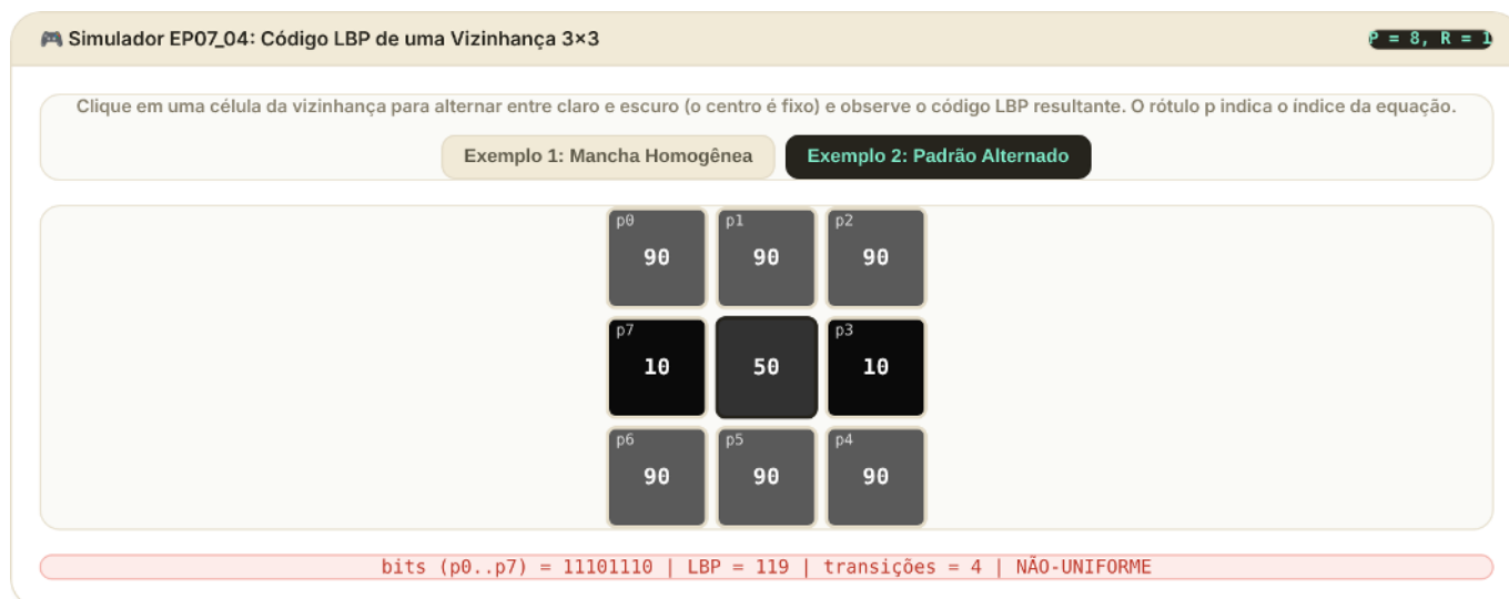
Figura 7.24: Simulador: Código LBP de uma Vizinhança 3 \times 3
