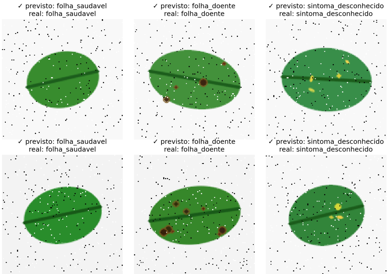
Figura 9.25: Predições da ResNet-18 ajustada em amostras de validação: rótulo previsto vs. rótulo real, com duas amostras por classe.
