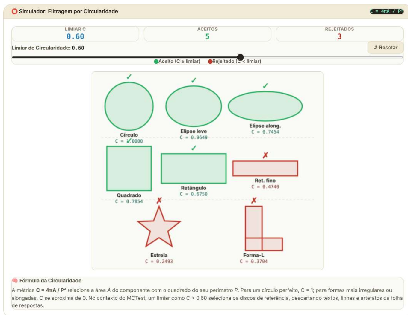
Figura 6.9: Simulador interativo de filtragem por circularidade: mova o slider para ajustar o limiar C e observe quais componentes são aceitos (verde) ou rejeitados (vermelho).
