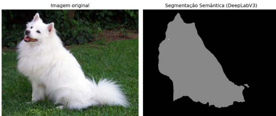
Figura 9.27: Mapa de segmentação semântica gerado pelo modelo DeepLabV3 pré-treinado: classificação pixel a pixel representada em matriz 2D exibida via mm.show .
