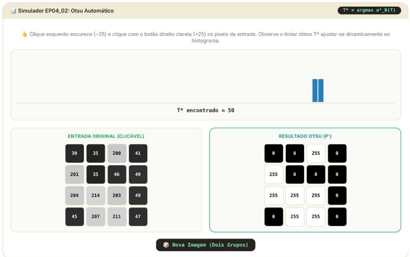
Figura 4.31: Simulador EP04_02: Limiarização Automática de Otsu ( T^* = \operatorname{argmax}_T \sigma^2_B(T) )
