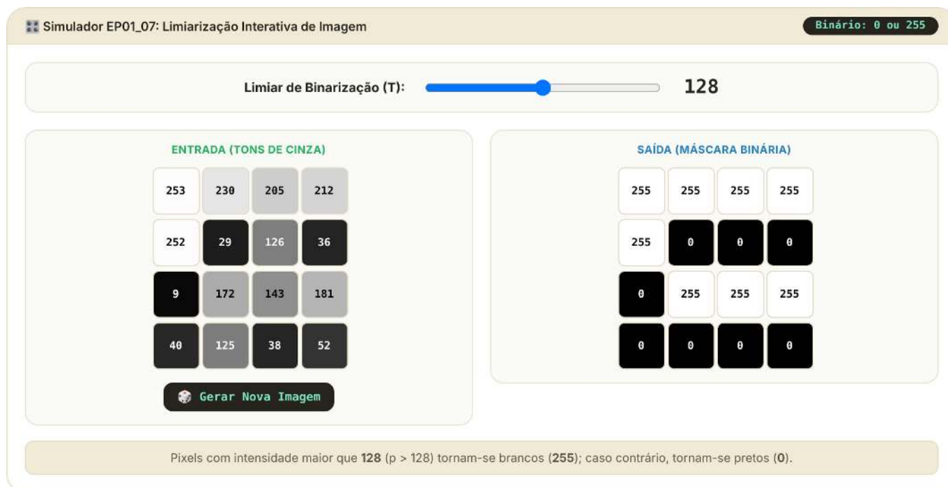
Figura 1.18: Simulador EP01_07: Limiarização Global Interativa (Binarização p > T )
