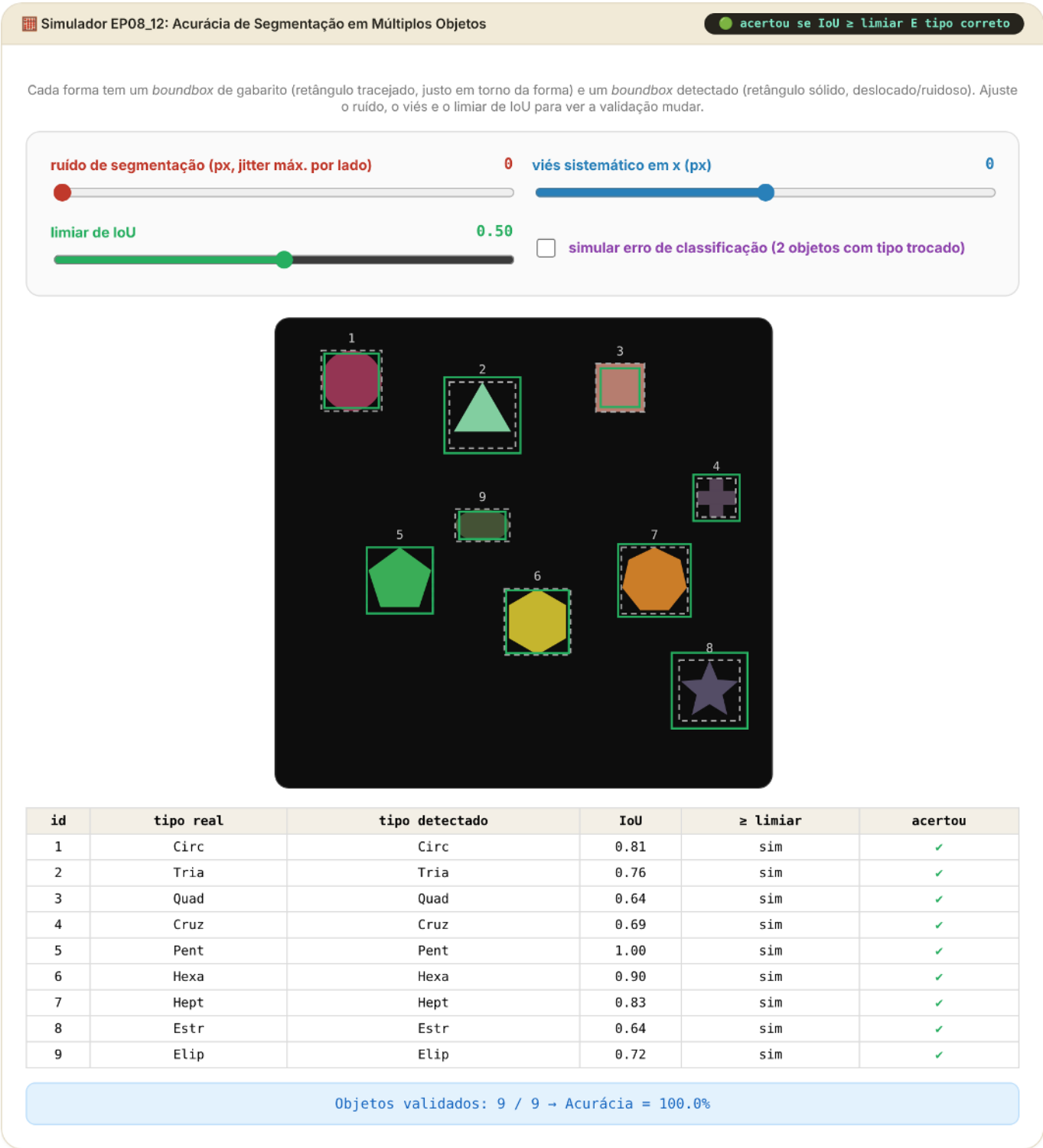
Figura 8.27: Simulador: Acurácia de Segmentação em Múltiplos Objetos (IoU)
