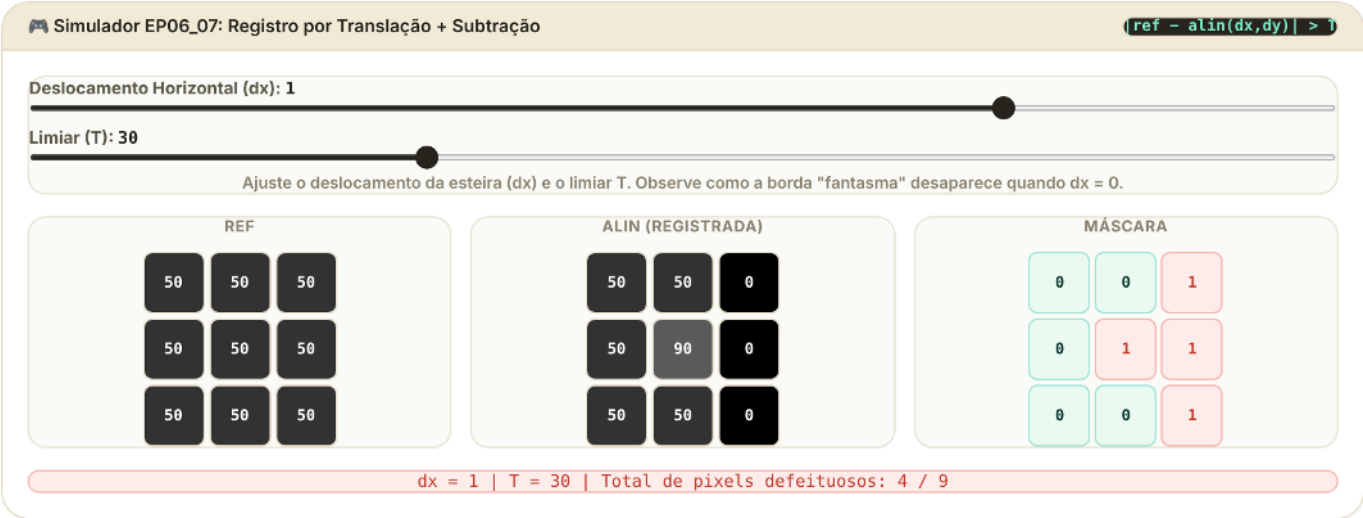
Figura 6.27: Simulador: Pipeline de Inspeção — Registro por Translação e Subtração
