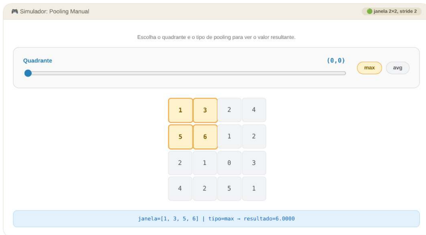
Figura 9.39: Simulador: Pooling Manual (máximo vs. média)
