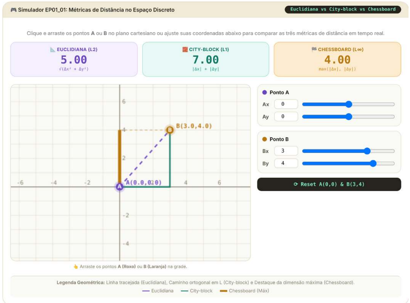
Figura 1.12: Simulador EP01_01: Distâncias Euclidiana, City-block e Chessboard
