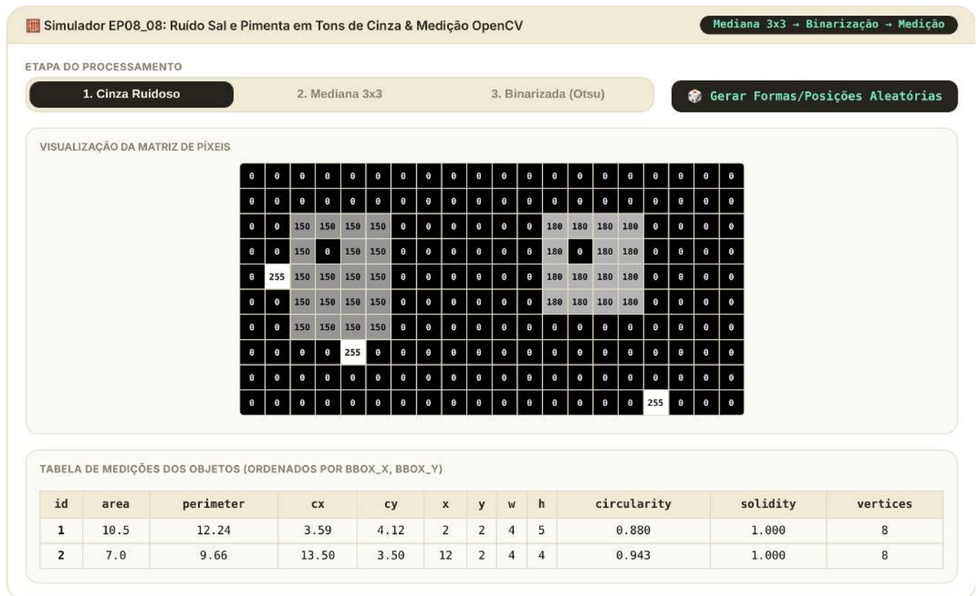
Figura 8.22: Simulador: Filtragem de Mediana em Tons de Cinza e Medição de Objetos OpenCV
