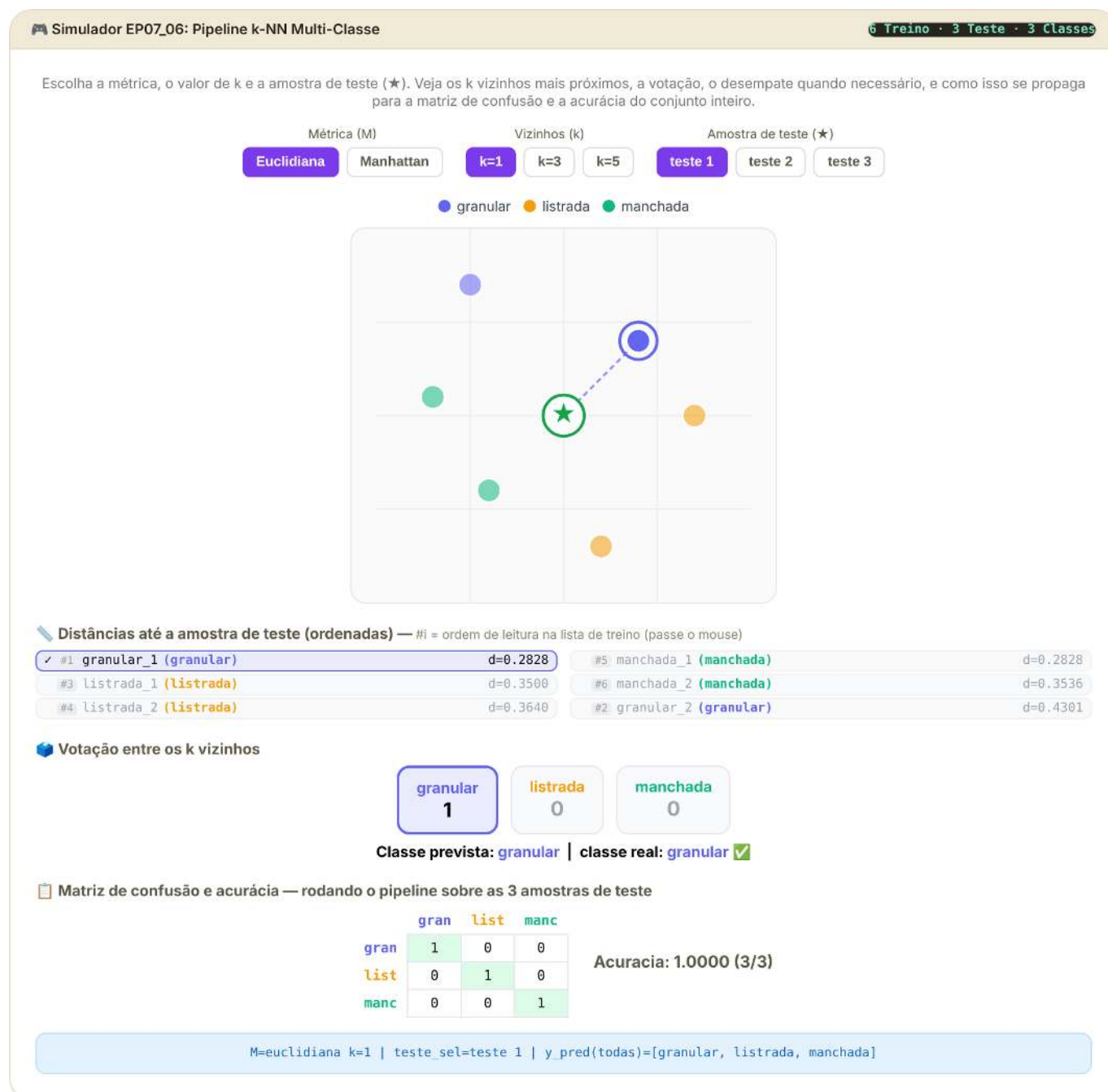
Figura 7.26: Simulador: Pipeline k-NN Multi-Classe (votacao, desempate e matriz de confusao)
