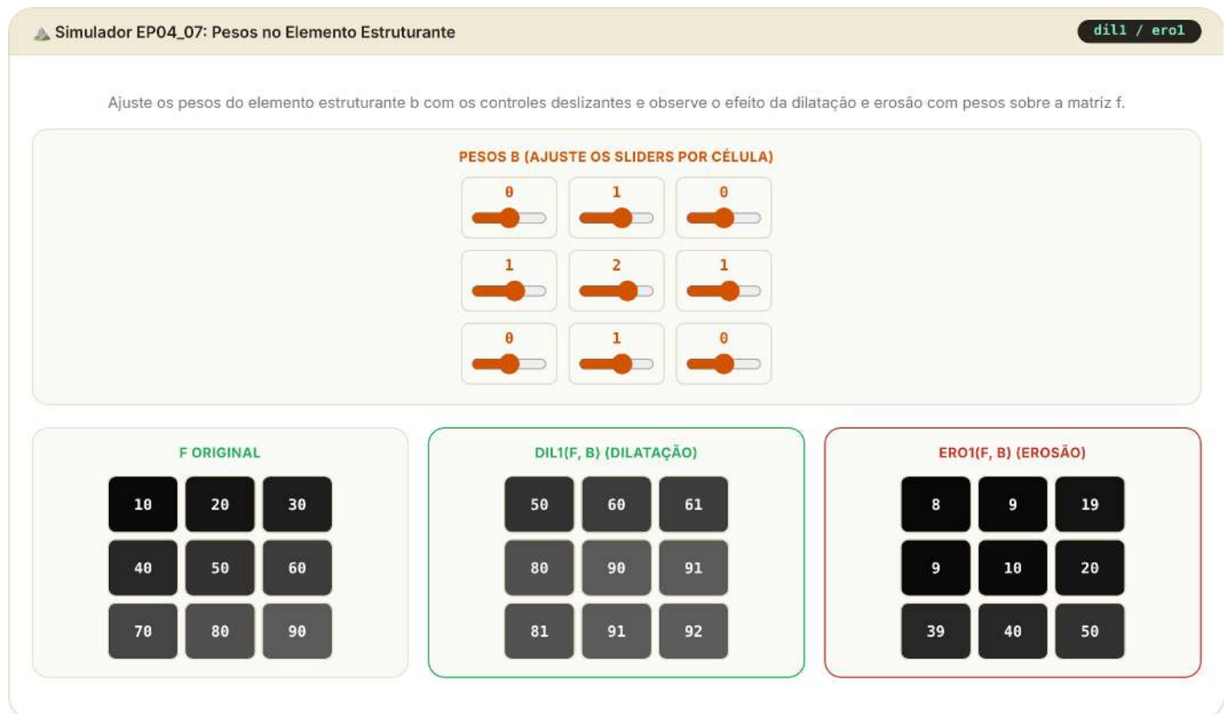
Figura 4.36: Simulador EP04_07: Dilatação e Erosão com Pesos (mm.dill1 / mm.ero1)
