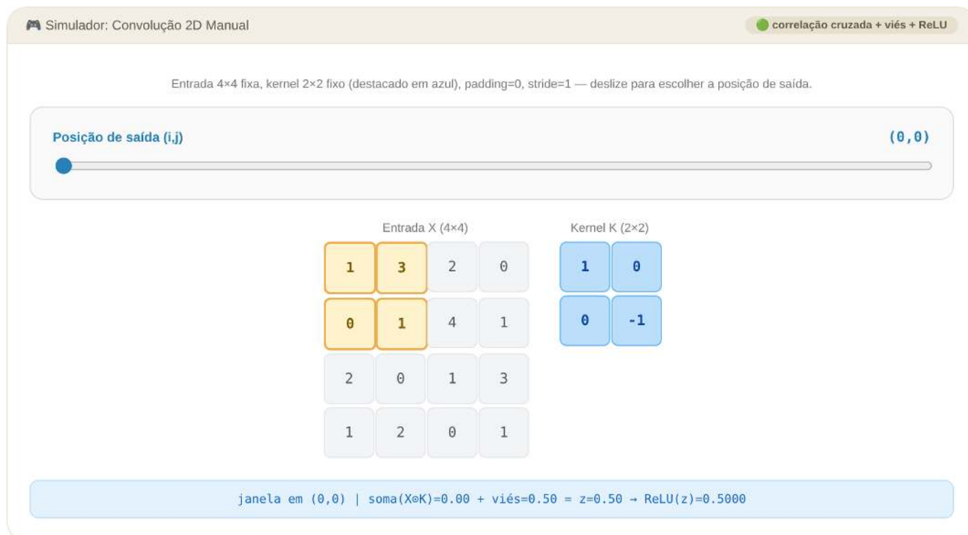
Figura 9.10: Simulador: Convolução 2D Manual (correlação cruzada + viés + ReLU)
