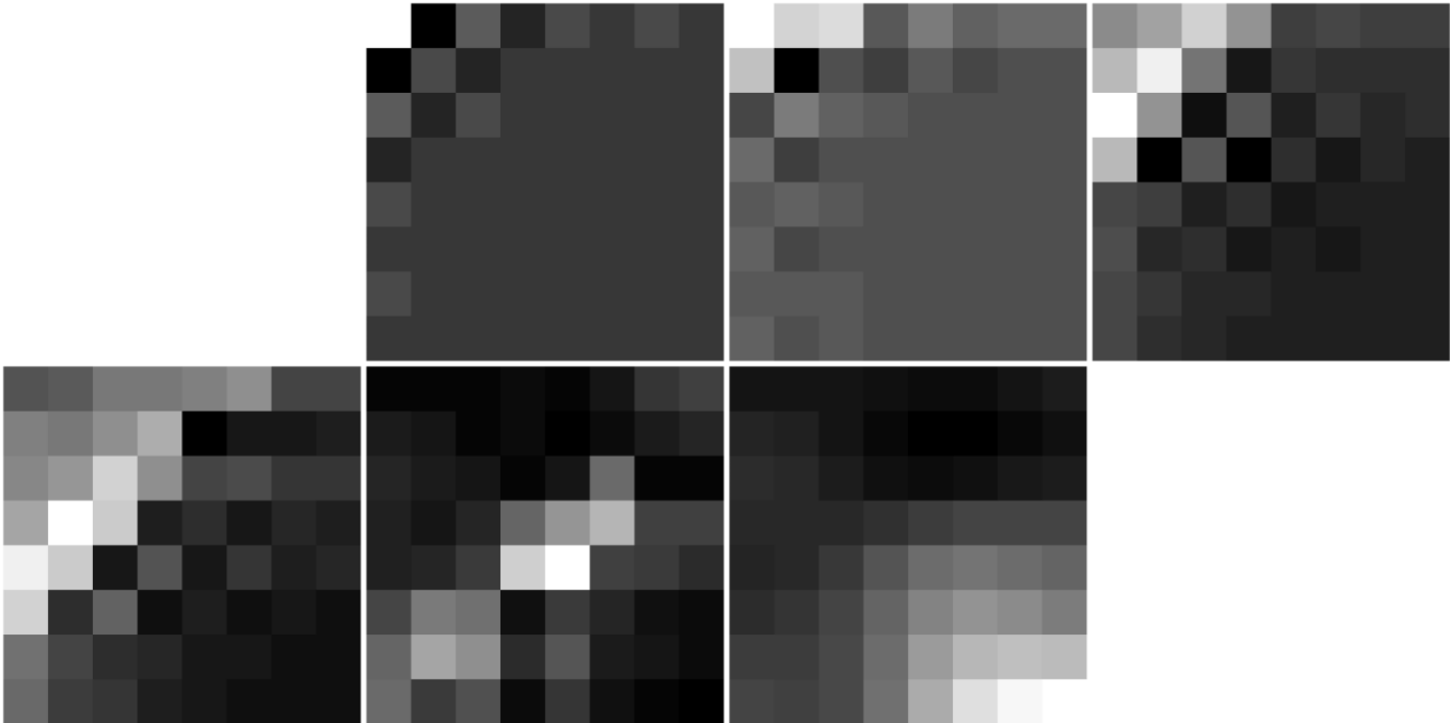
Figure 5.24: DCT 2D em bloco 8x8: coeficientes e reconstrução progressiva.
