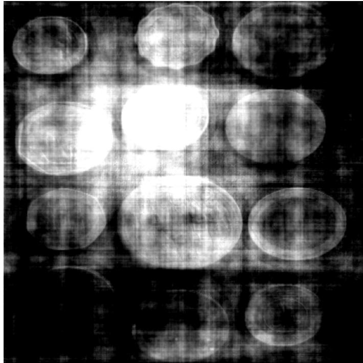
Mag(B) + Fase(A)
