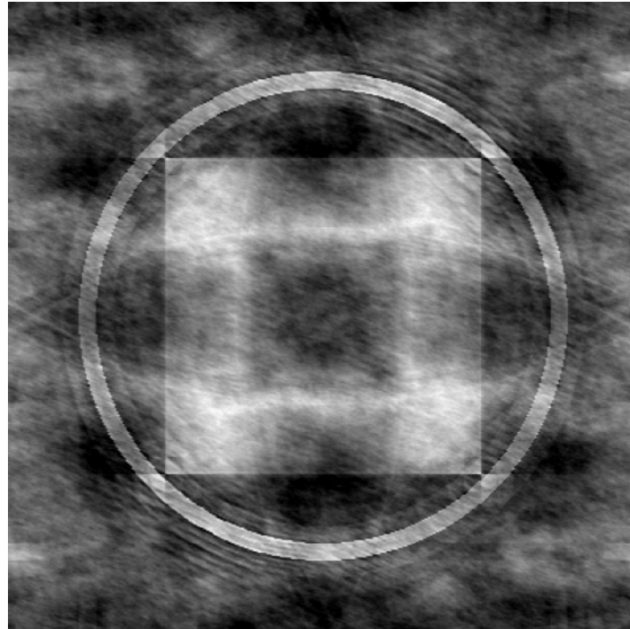
Mag(A) + Fase(B)
