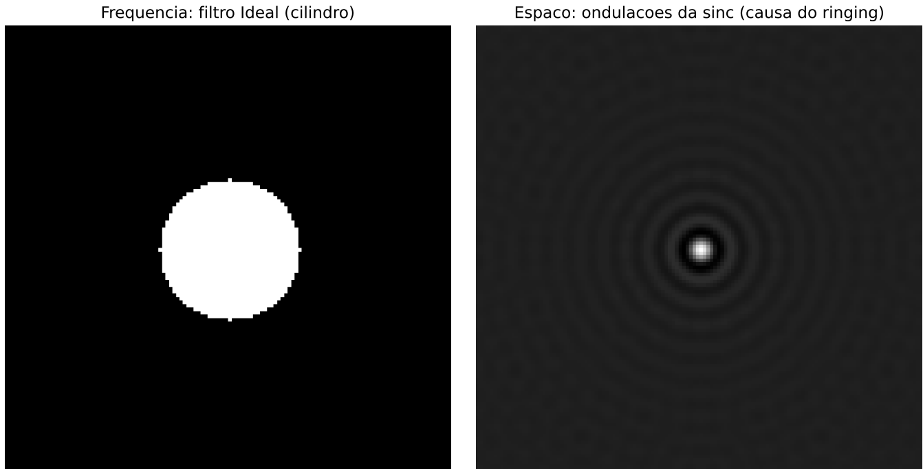
Figure 5.10: A Dualidade Perigosa: o corte abrupto na Frequência (cilindro Ideal) vira obrigatoriamente uma sinc no espaço. Suas ondulações causam o ringing fantasma nas bordas da imagem.
