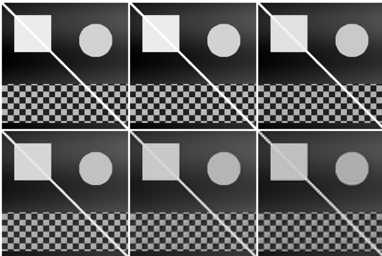
Figure 5.22: Reconstituição wavelet com limiarização de coeficientes ( hard thresholding ): à medida que o limiar aumenta, mais detalhes são zerados, produzindo imagens progressivamente mais suaves. Métrica PSNR quantifica a perda de qualidade sobre o padrão sintético.
