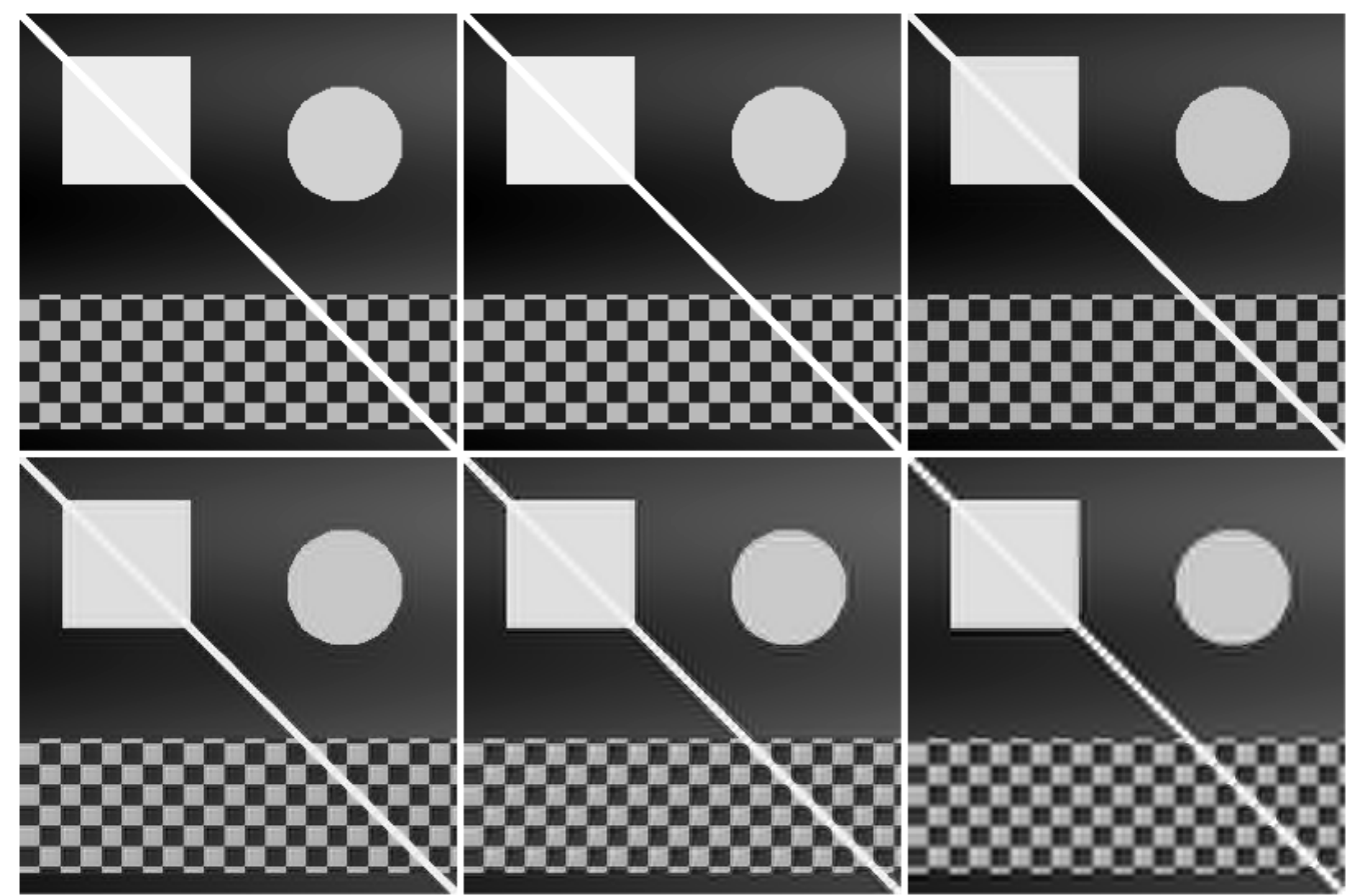
Figura 5.22: Ricostruzione wavelet con limitazione di coefficienti ( hard thresholding ): a misura che il limite aumenta, più dettagli sono azzerati, producendo immagini progressivamente più lisce. Metrica PSNR quantifica la perdita di qualità rispetto al modello sintetico.
