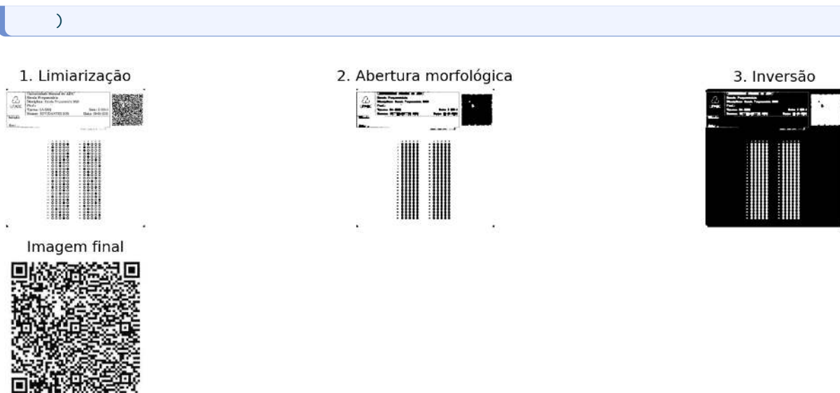
Figura 6.8: Pipeline de processamento do QRCode : limiarização, abertura morfológica, inversão e recorte final para decodificação.
